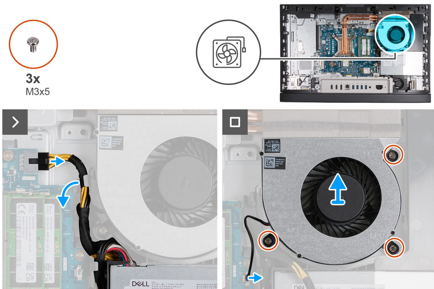
Figura 48. Rimozione della ventola
