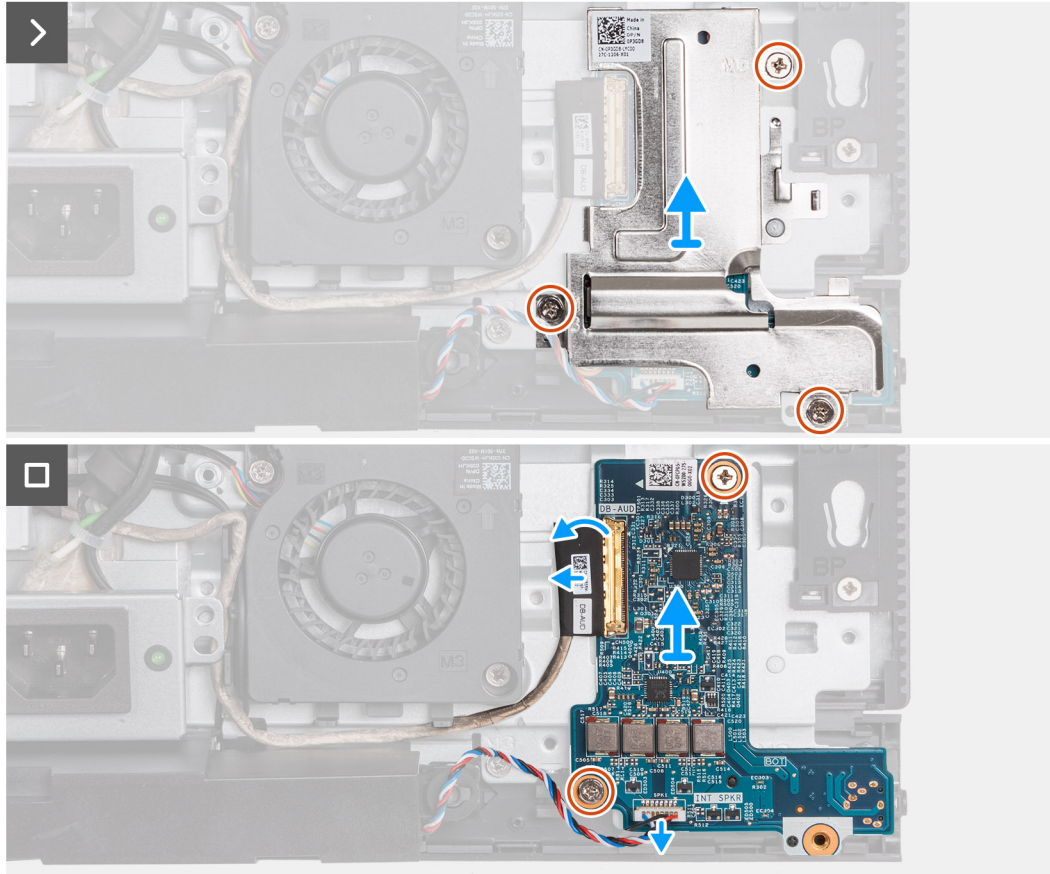
Figura 74. Rimozione della scheda audio
