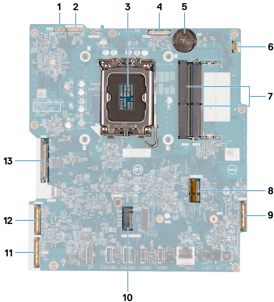
Figura 116. Callout della scheda di sistema
