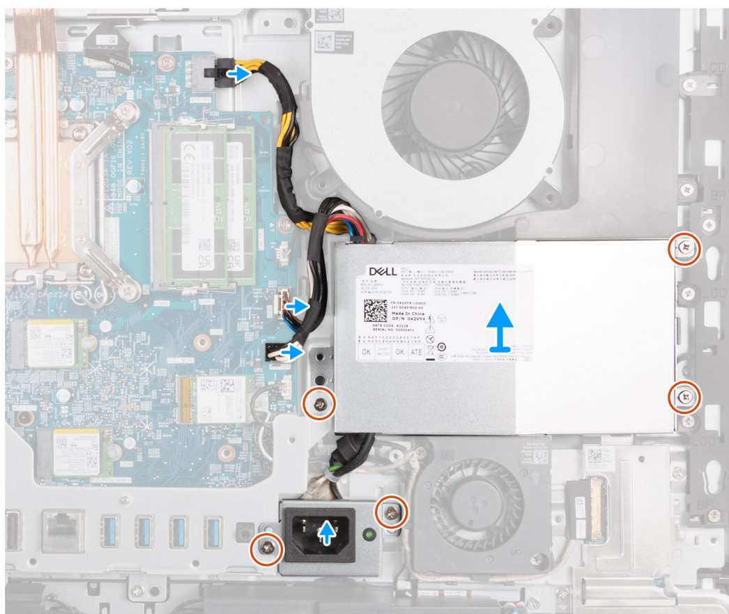
Figura 50. Rimozione dell'unità di alimentazione
