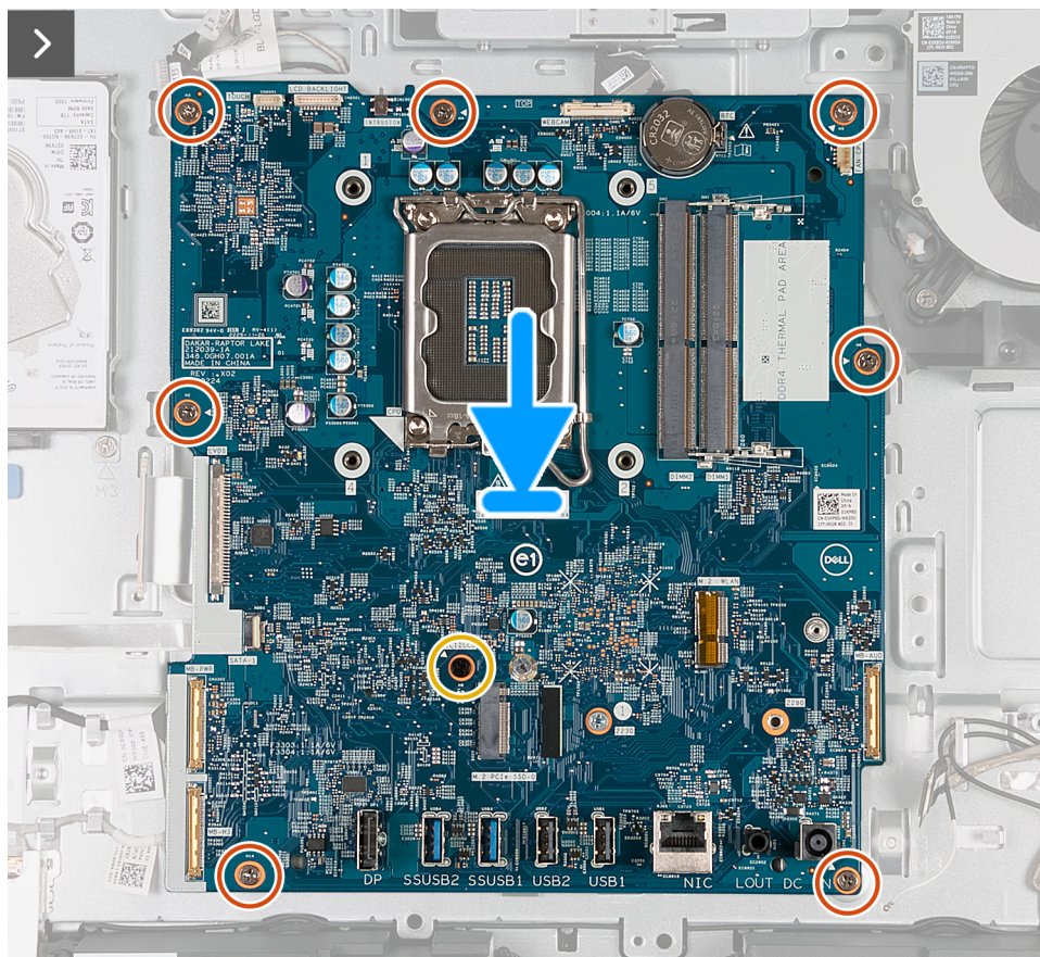
Figura 117. Installazione della scheda di sistema
