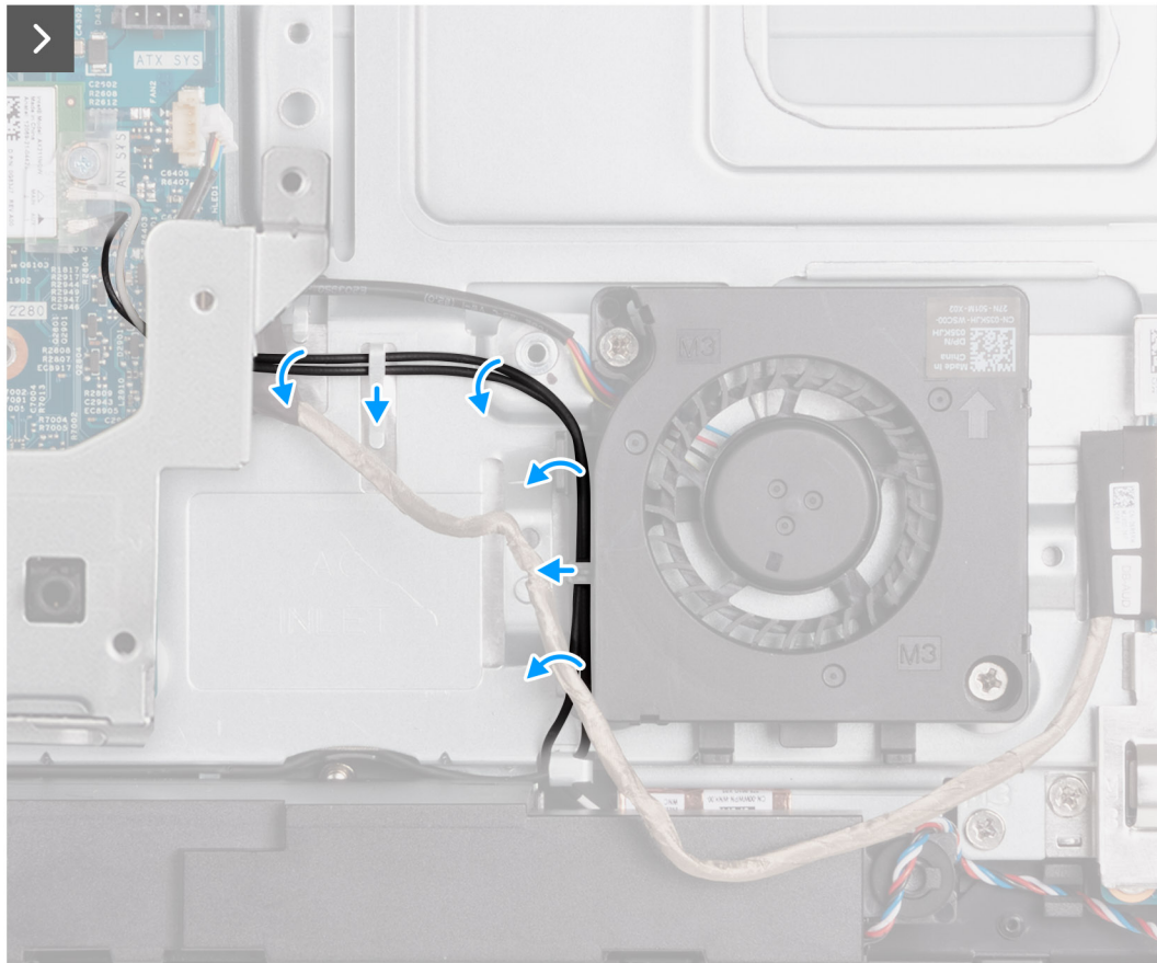
Figura 53. Rimozione della ventola di alimentazione
