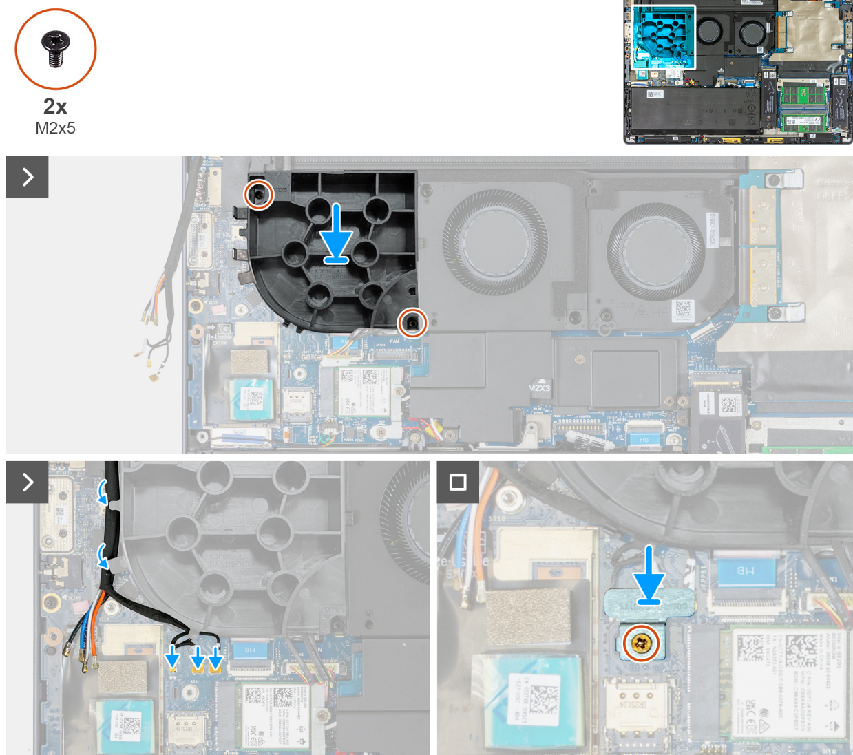
Figura 60. Installazione della ventola fittizia
