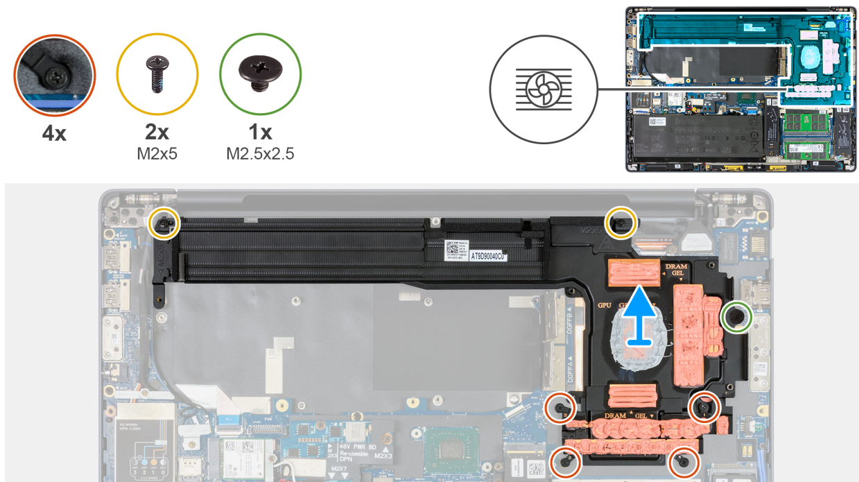
Figura 75. Rimozione del dissipatore di calore per computer forniti con scheda grafica dedicata
