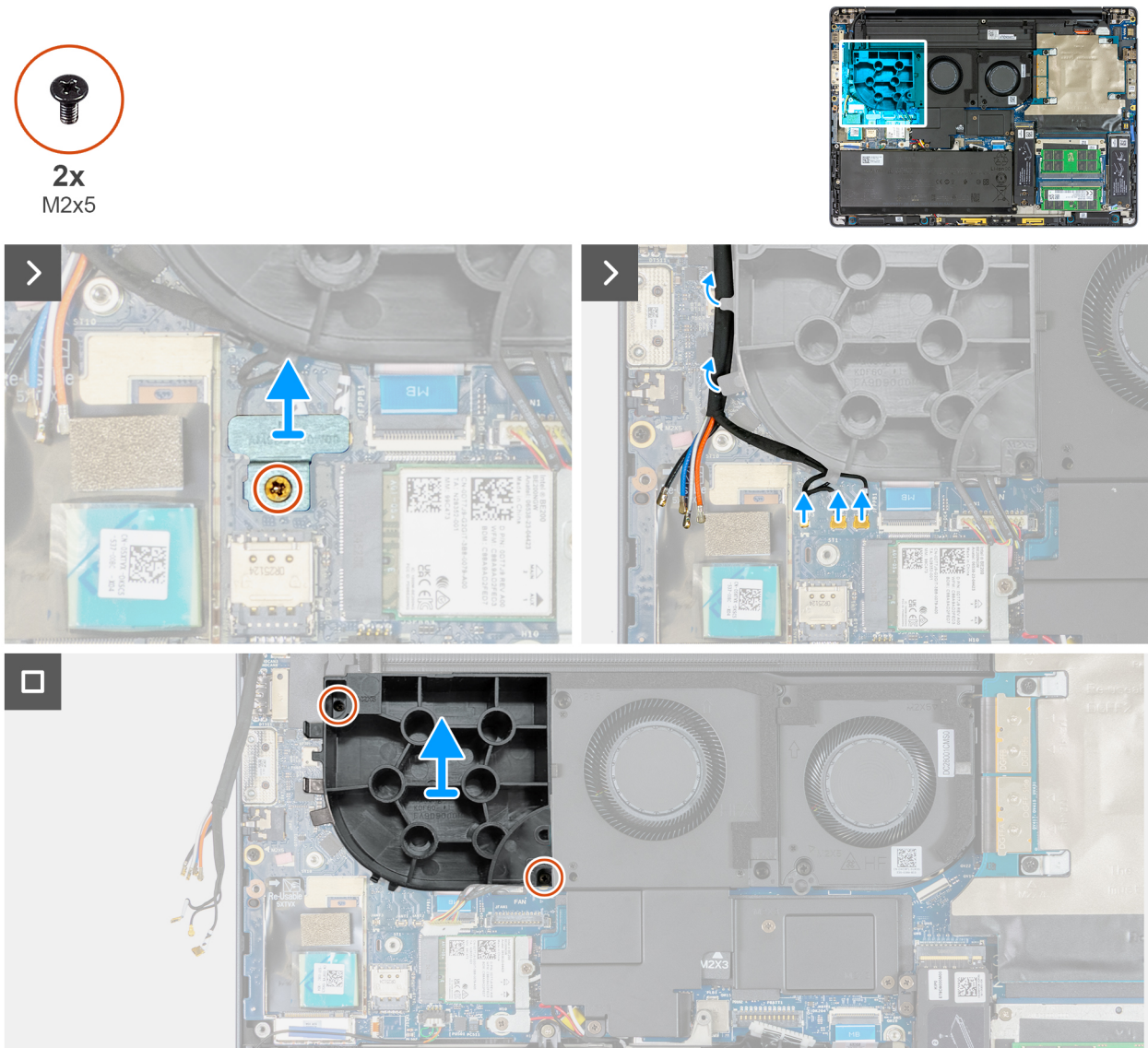
Figura 59. Rimozione della ventola fittizia
