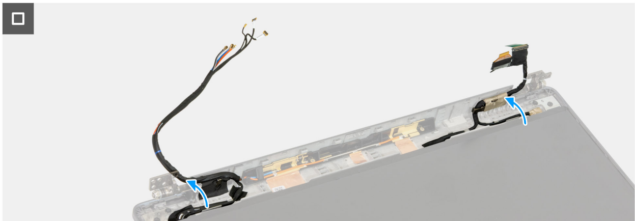
Figura 100. Installazione delle cerniere del display
