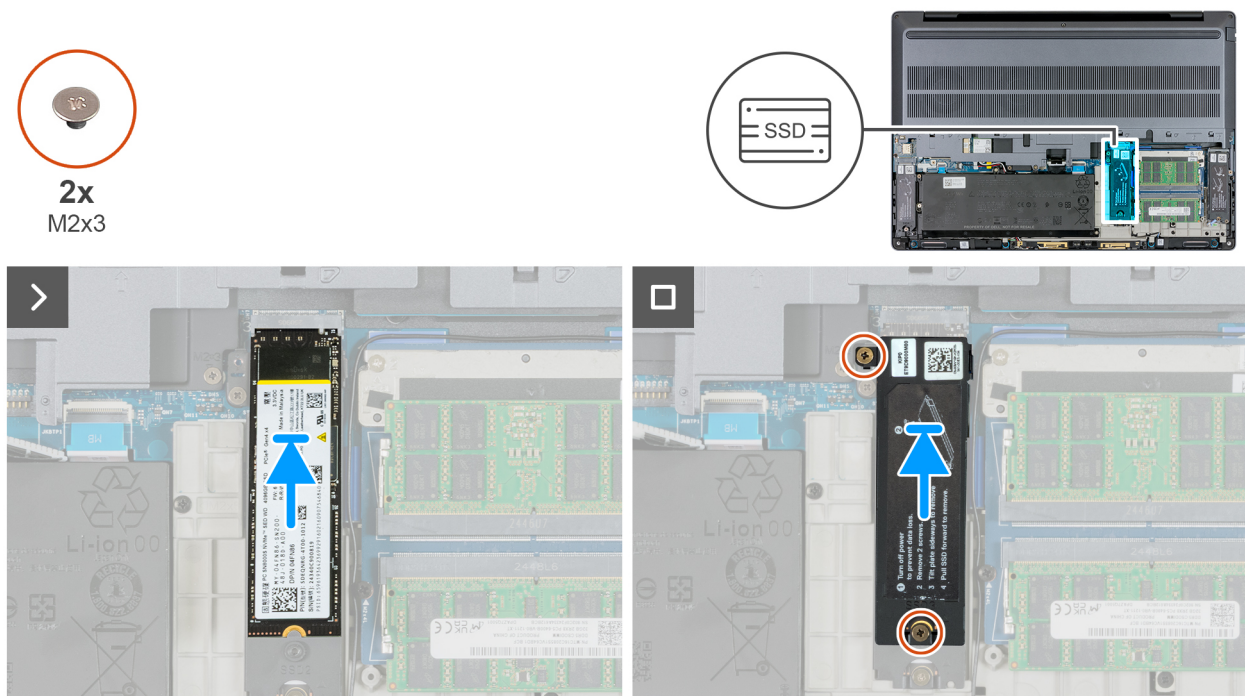
Figura 37. Installazione dell'SSD M.2 2280 nello slot 3 (SSD3)
