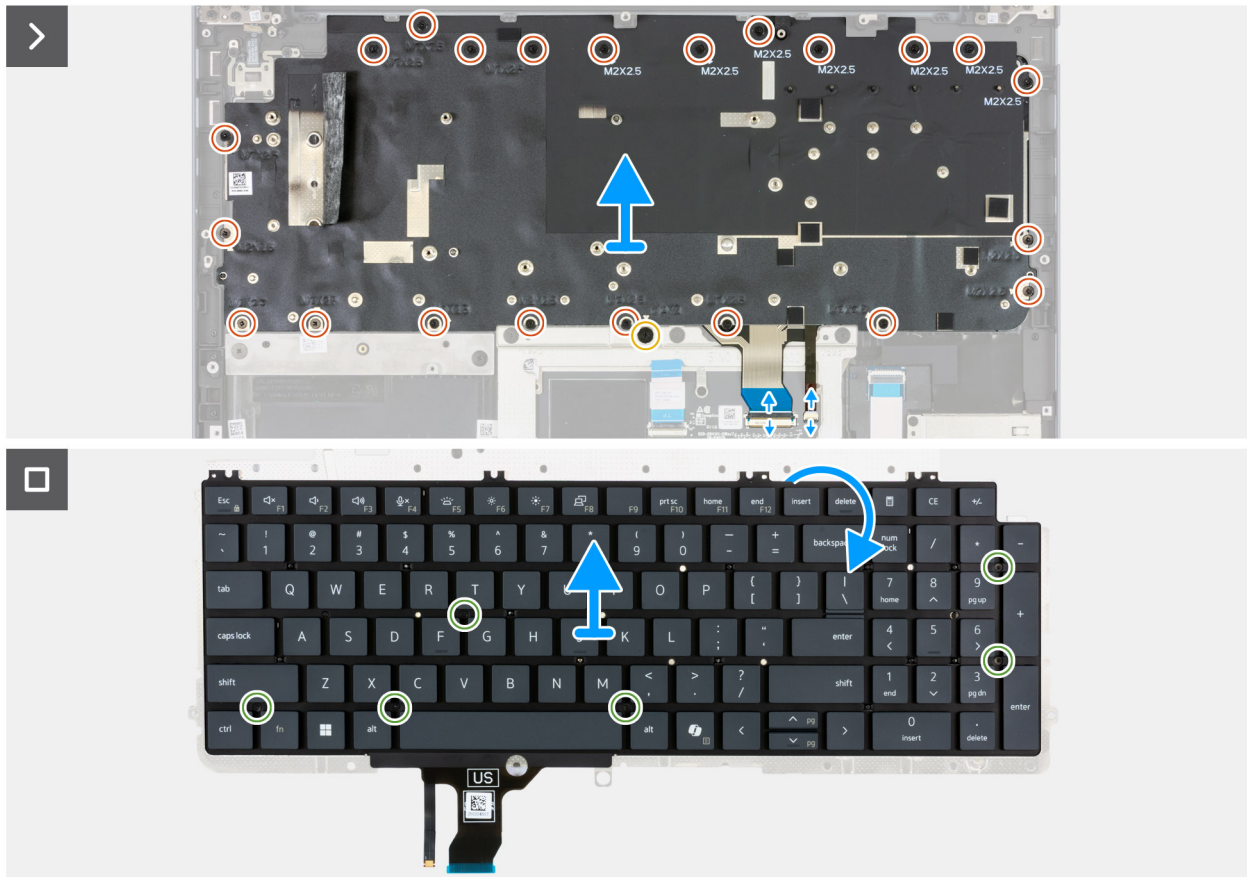
Figura 121. Rimozione della tastiera
