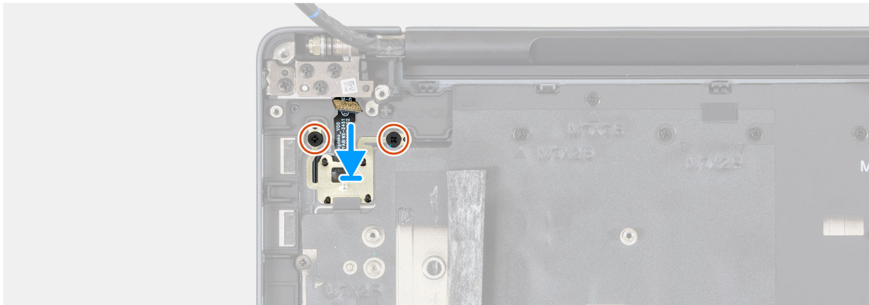
Figura 130. Installazione del pulsante di accensione
