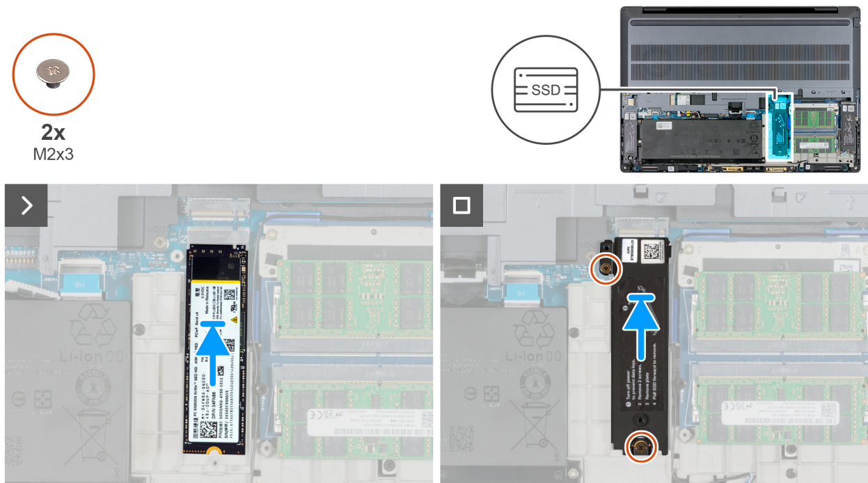
Figura 39. Installazione dell'SSD M.2 2280 nello slot 2 (SSD2)
