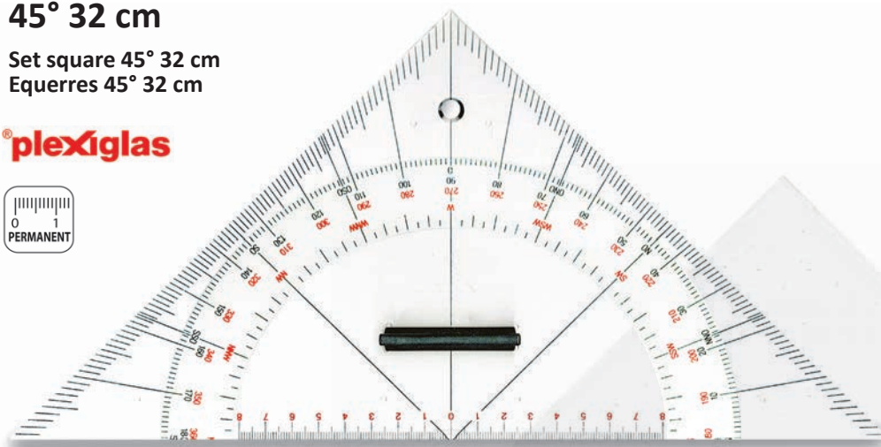
Ref. 418 Con pomolo, millimetrata con linea di fede sul bordo. With grip, graduated with hypotenuse scale on the edge. Avec poignée et graduation hypotenuse sur le bord.
