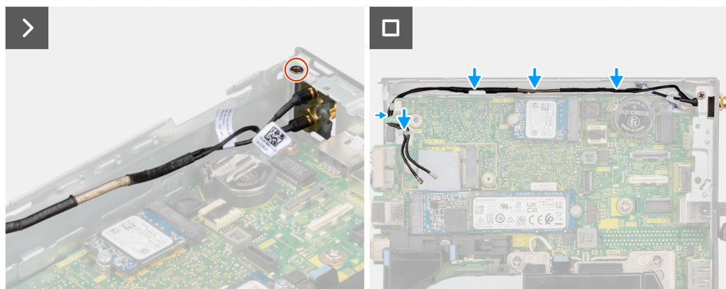
Figura 55. Installazione dell'antenna SMA (posizione 3)
