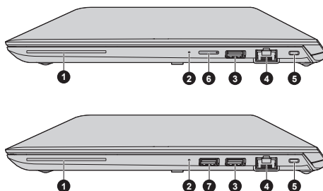
Figura 3-3 Lato destro del computer
