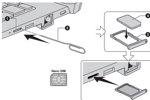
Figura 4-5 Installazione della scheda SIM
