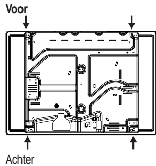
Stand haak voor keukenblad H=40mm
