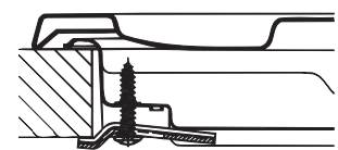
Posição do gancho para H=30mm
