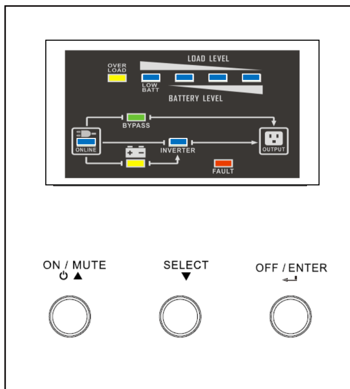
Figura 2 - Pannello Frontale
