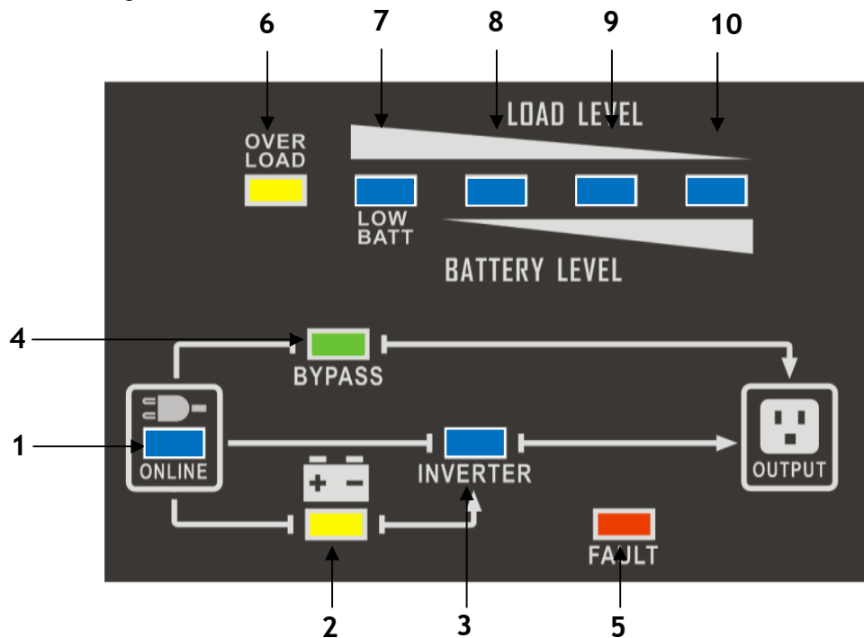
Figura 3 - Pannello Led
