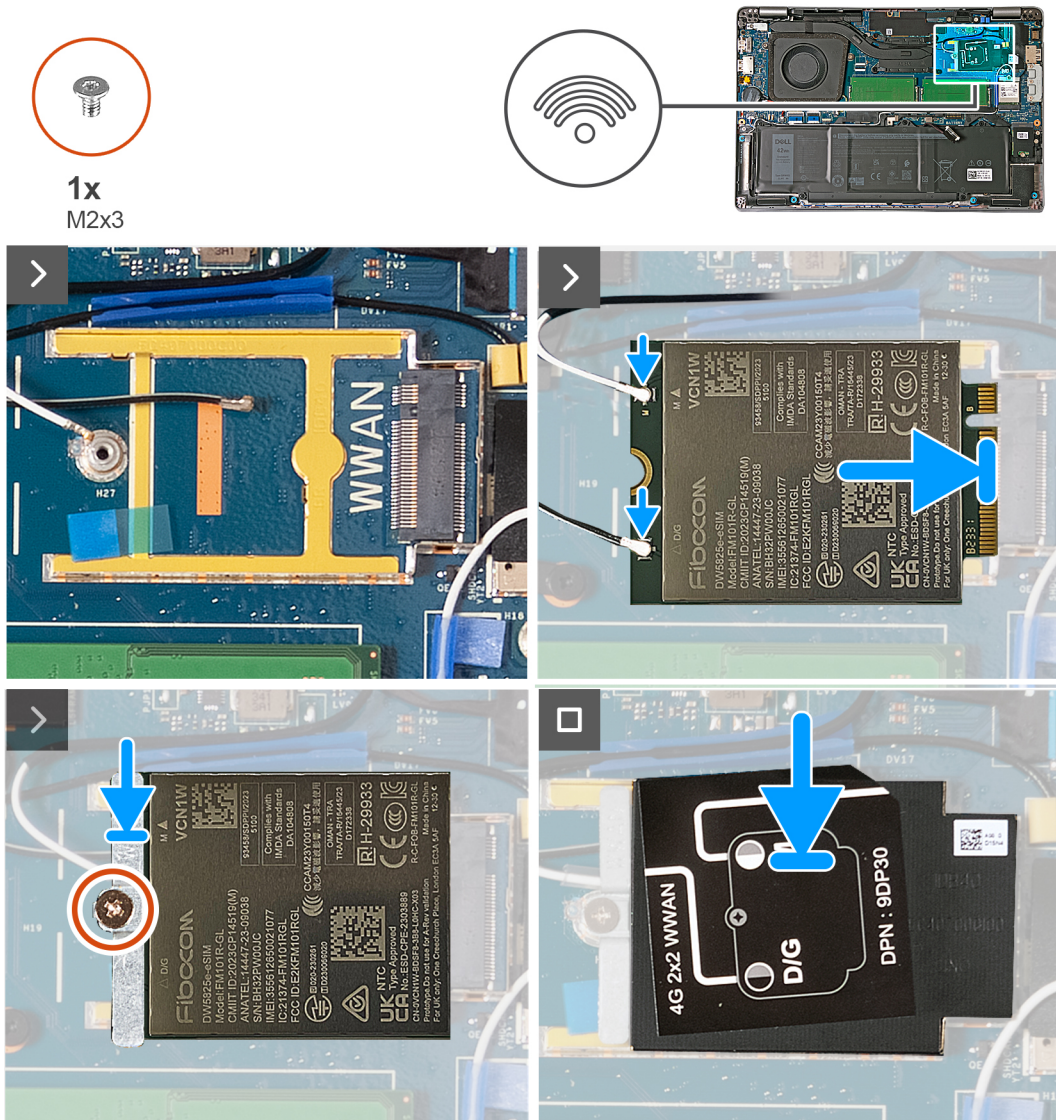
Figura 22. Installazione della scheda WWAN - Per computer forniti con scheda 4G
