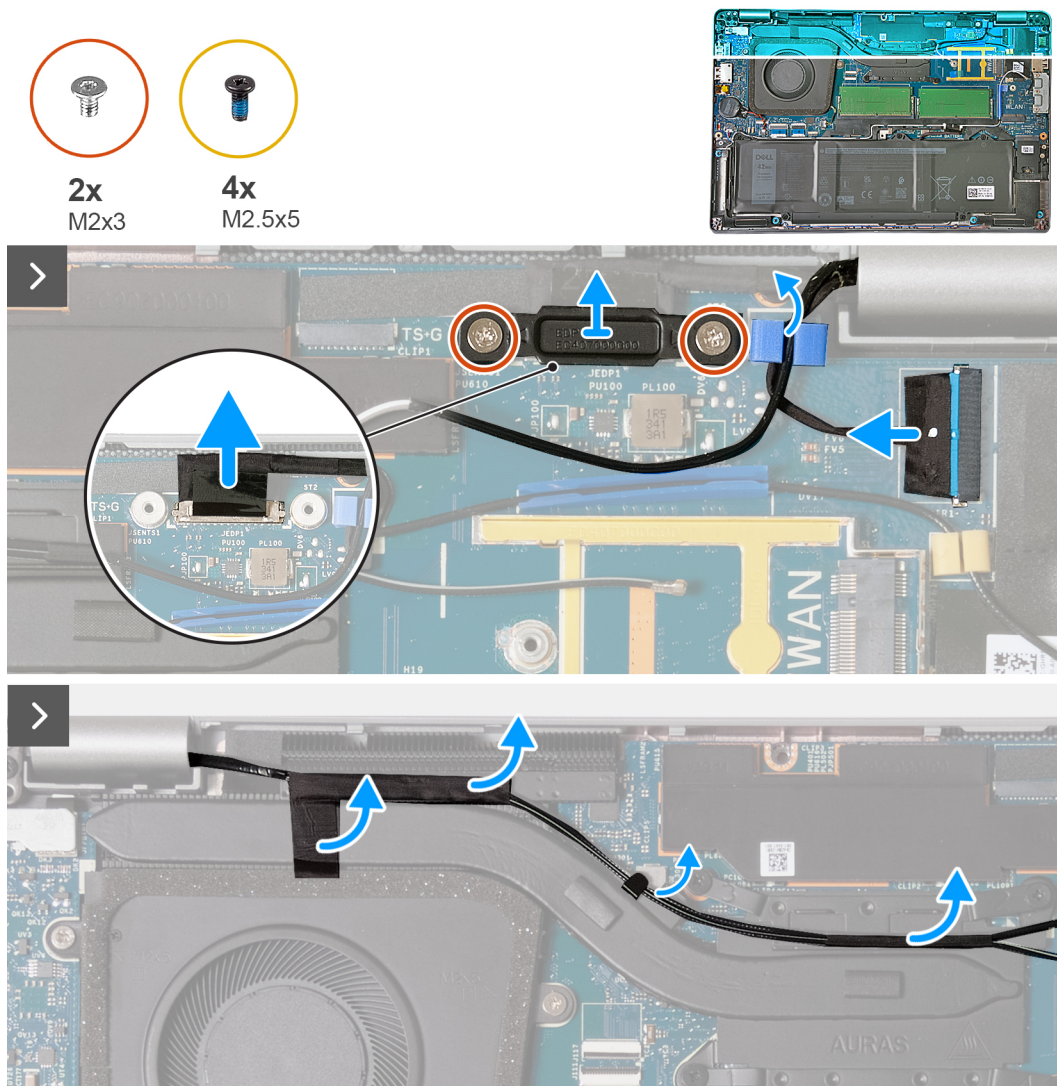
Figura 43. Rimozione del gruppo del display - Per i computer forniti con scheda 4G
