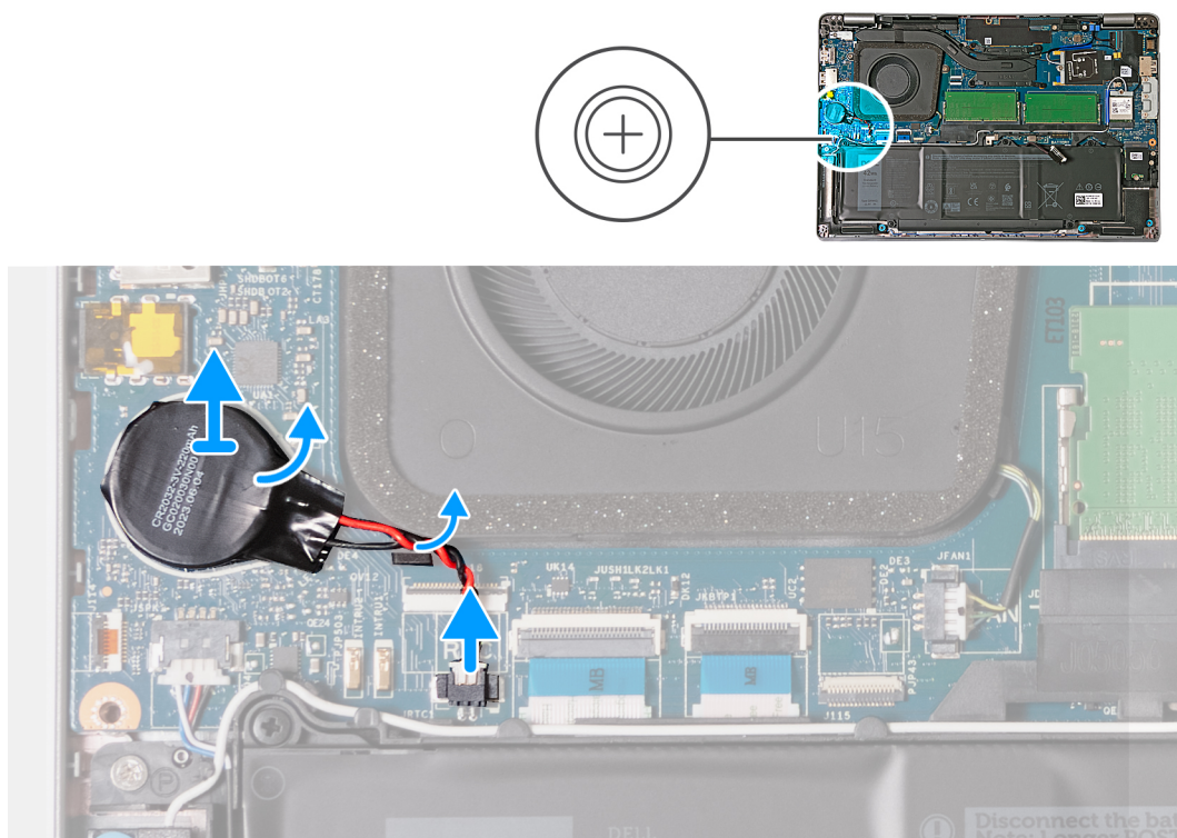
Figura 28. Rimozione della batteria a bottone
