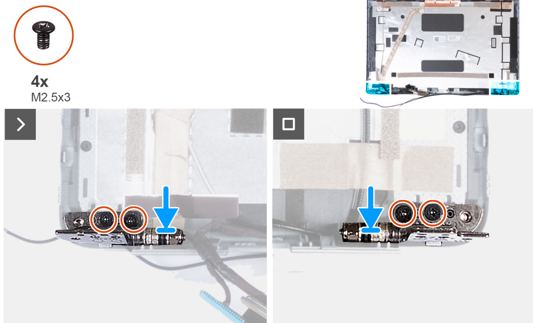
Figura 61. Installazione delle cerniere del display
