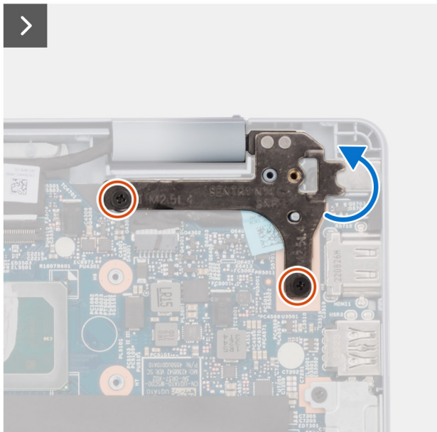
Figura 46. Rimozione della porta dell'adattatore per l'alimentazione
