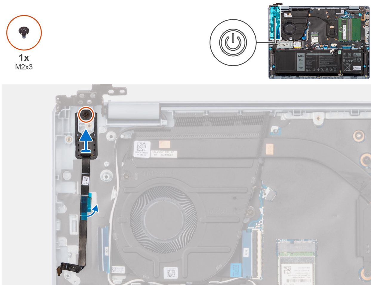
Figura 54. Immagine: Rimozione del pulsante di accensione
