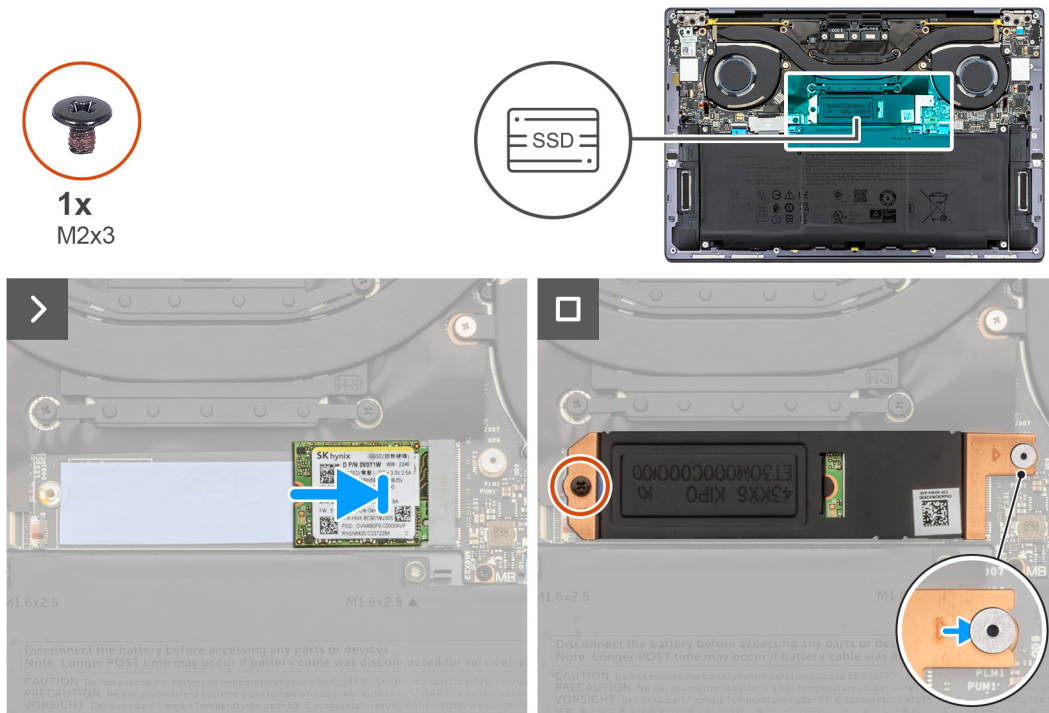
Figura 21. Installazione dell'SSD M.2 2230
