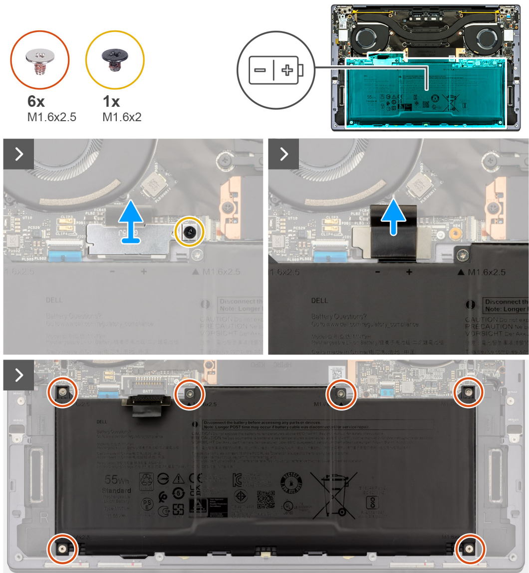
Figura 14. Rimozione della batteria
