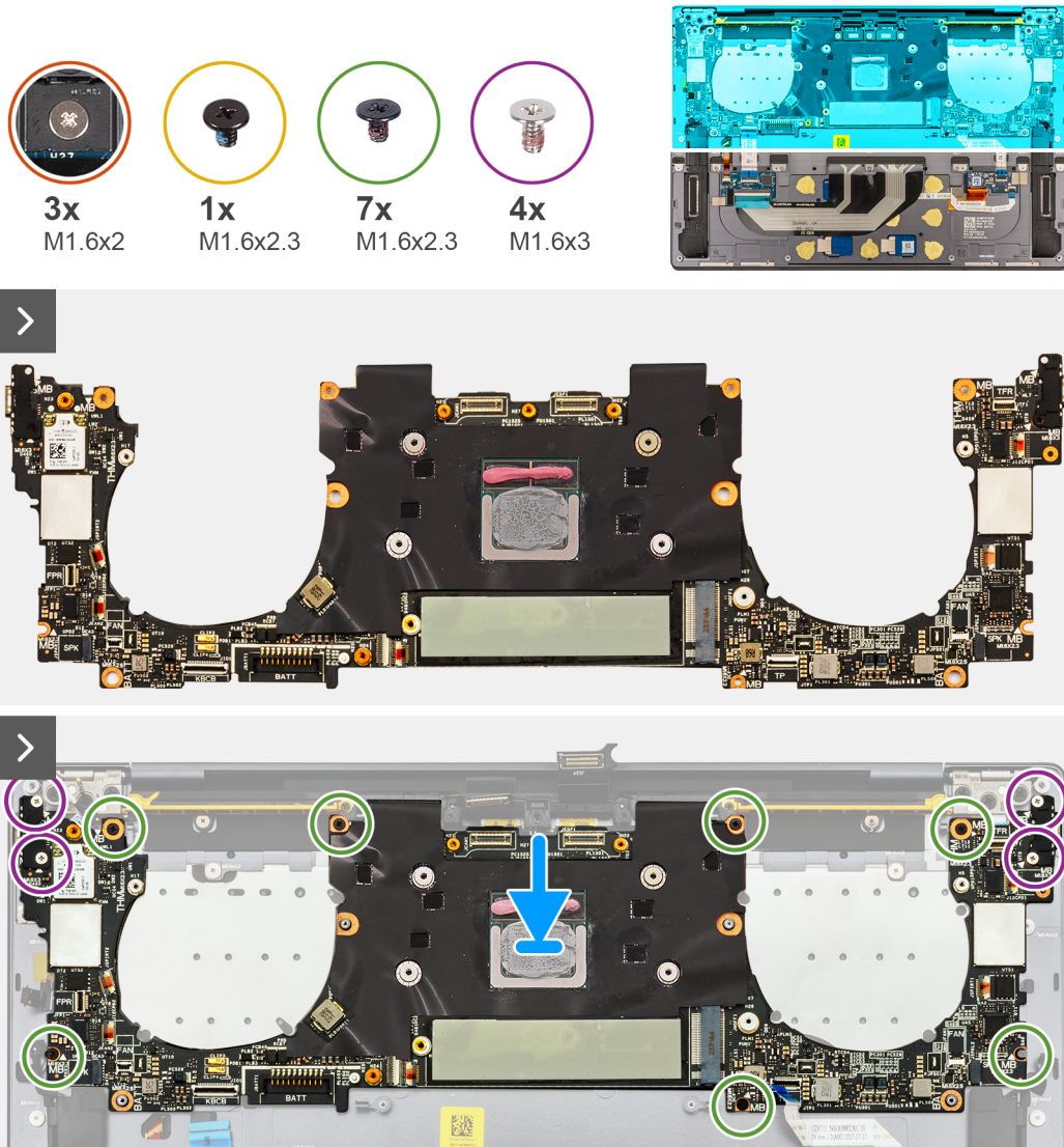
Figura 40. Installazione della scheda di sistema
