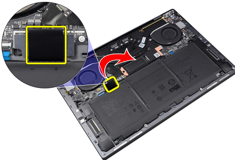
Figura 16. Rimozione della staffa del connettore della batteria
