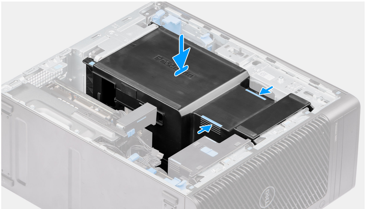
Figura 15. Installazione del manicotto dell'aria
