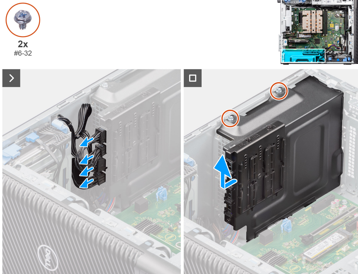
Figura 46. Rimozione del coperchio dell'unità di alimentazione
