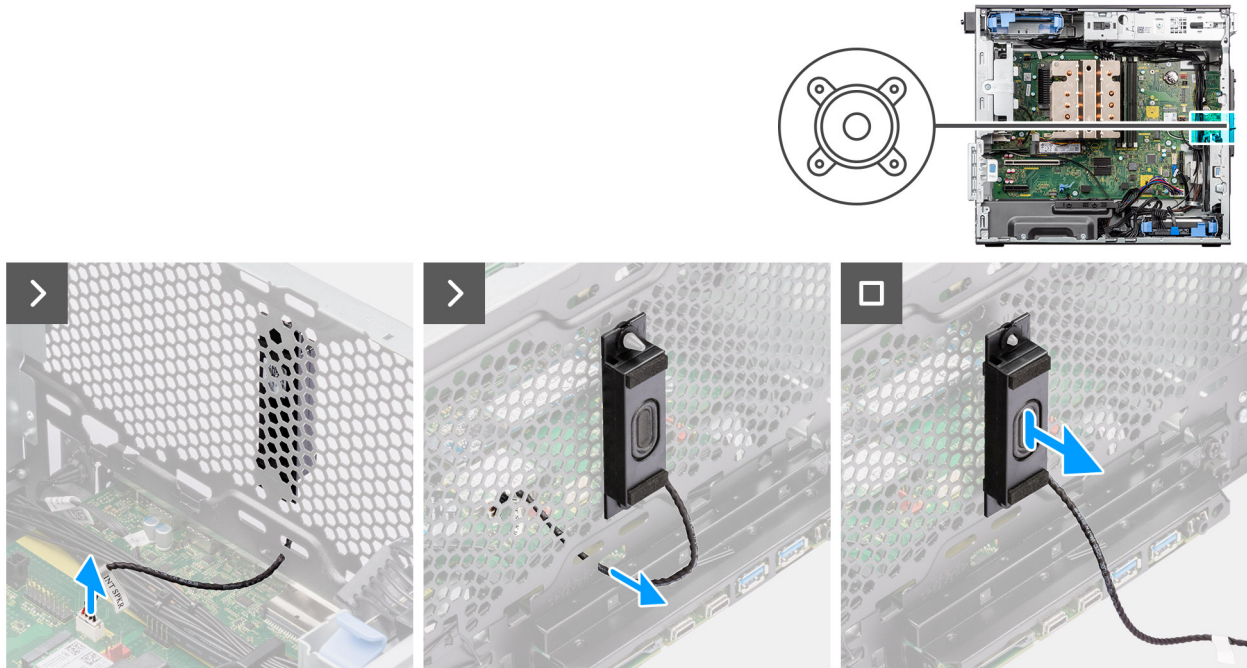
Figura 72. Rimozione dell'altoparlante interno
