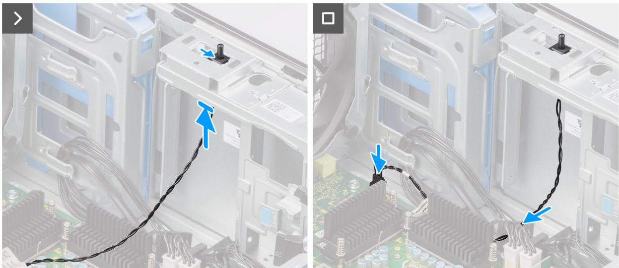
Figura 71. Installazione dell'interruttore di apertura
