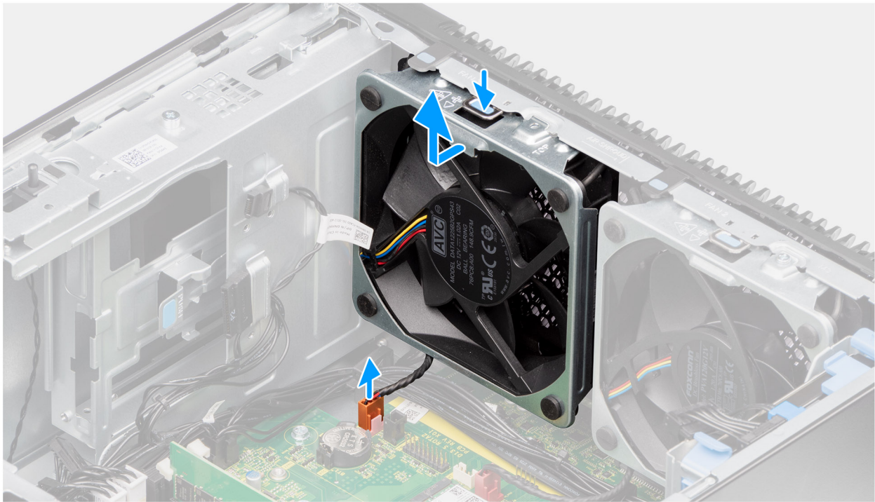
Figura 61. Ventola anteriore 2
