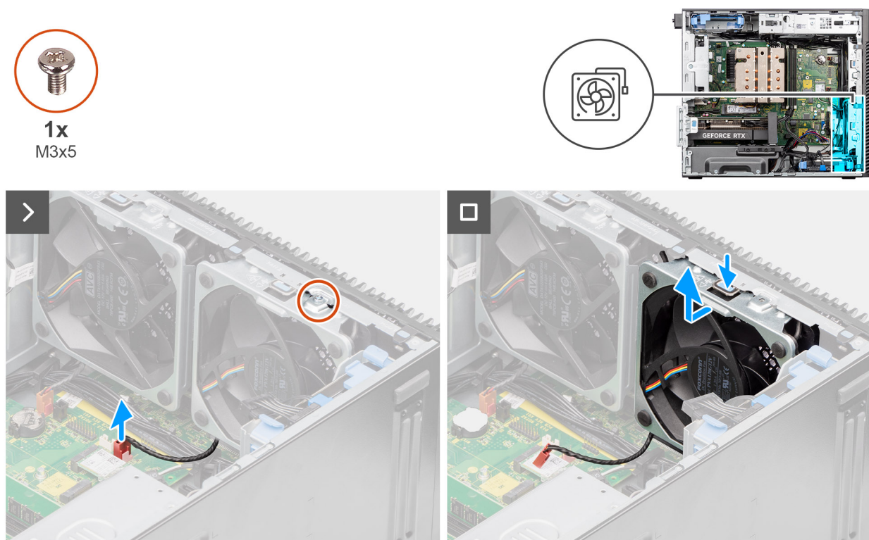
Figura 60. Ventola anteriore 1
