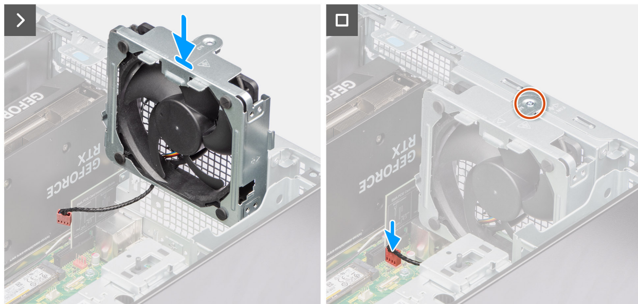
Figura 67. Installazione della ventola posteriore (PSU da 1.000 W)
