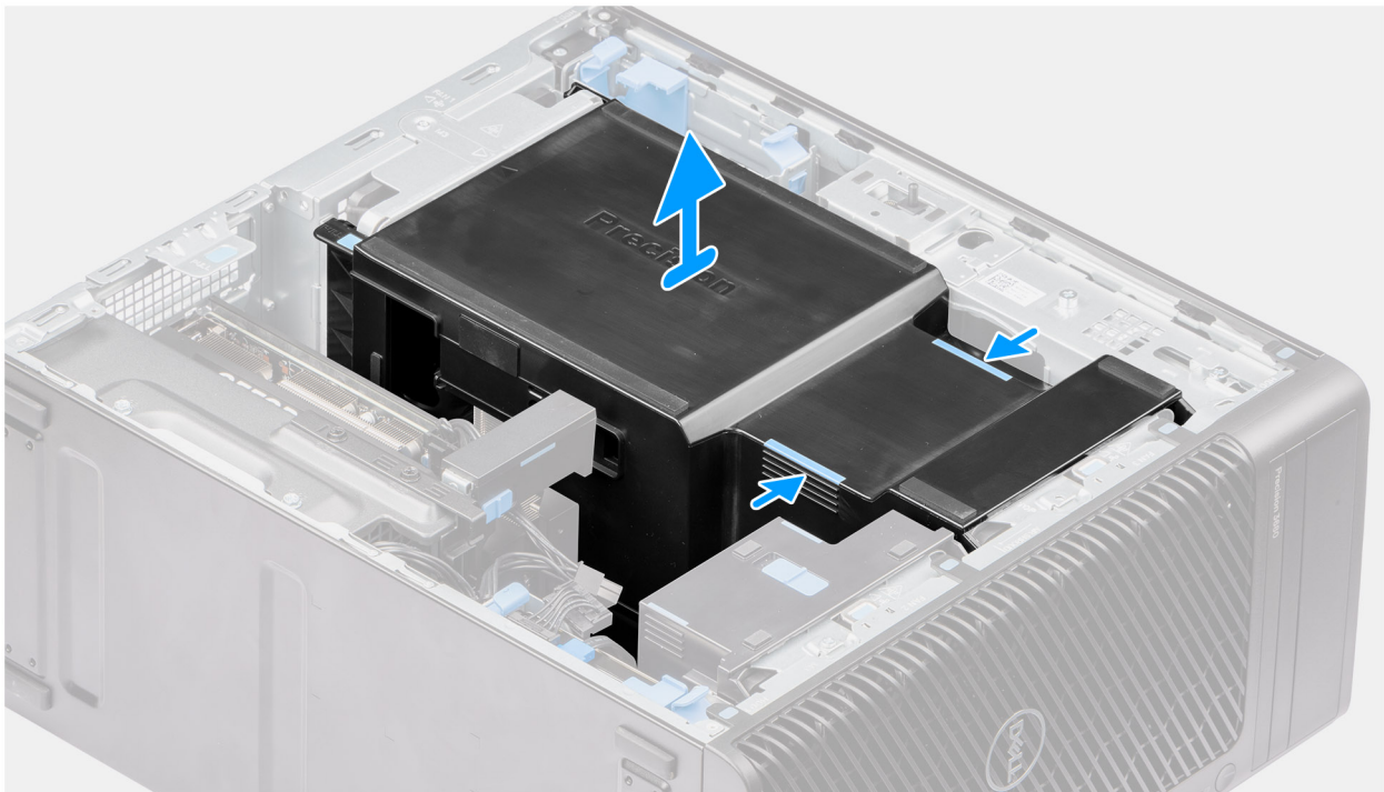
Figura 14. Rimozione del manicotto dell'aria
