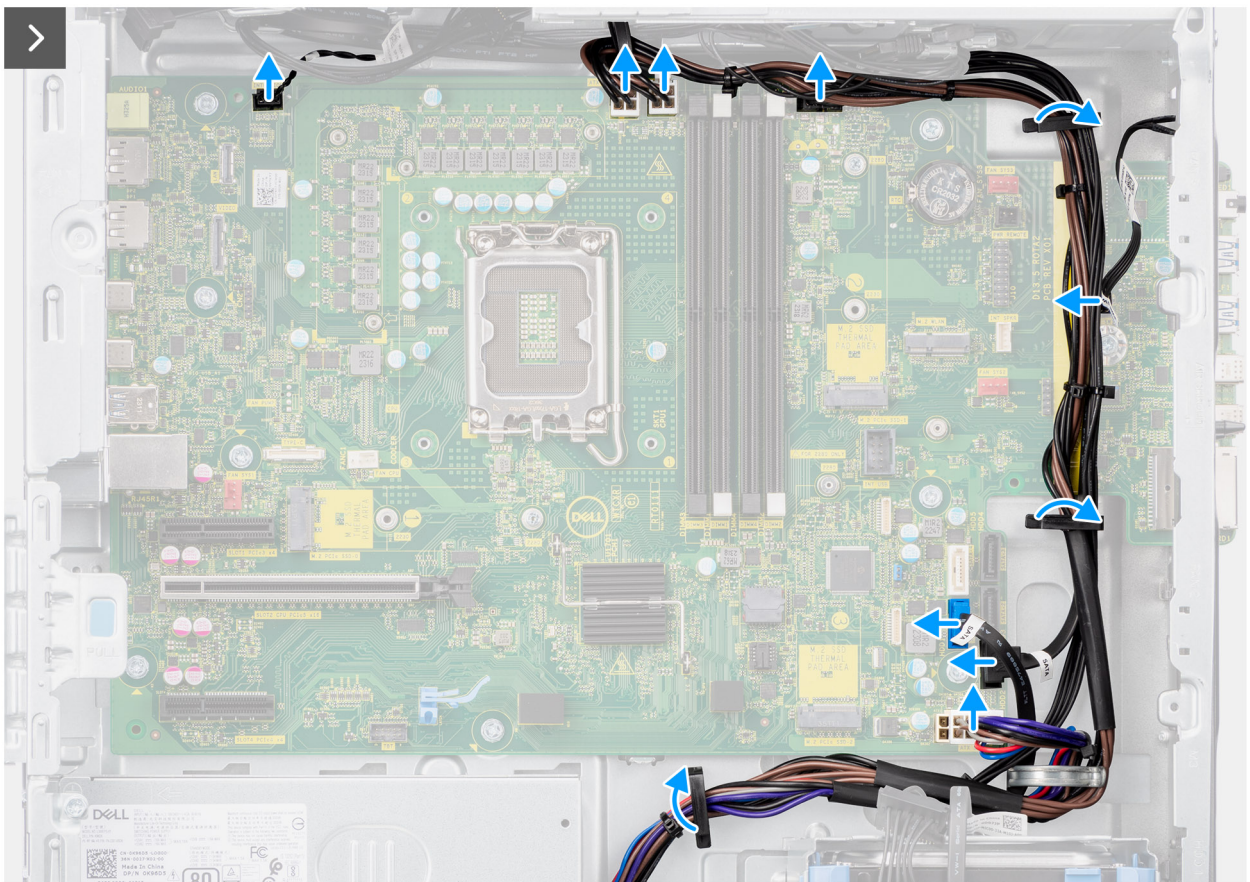
Figura 76. Rimozione della scheda di sistema
