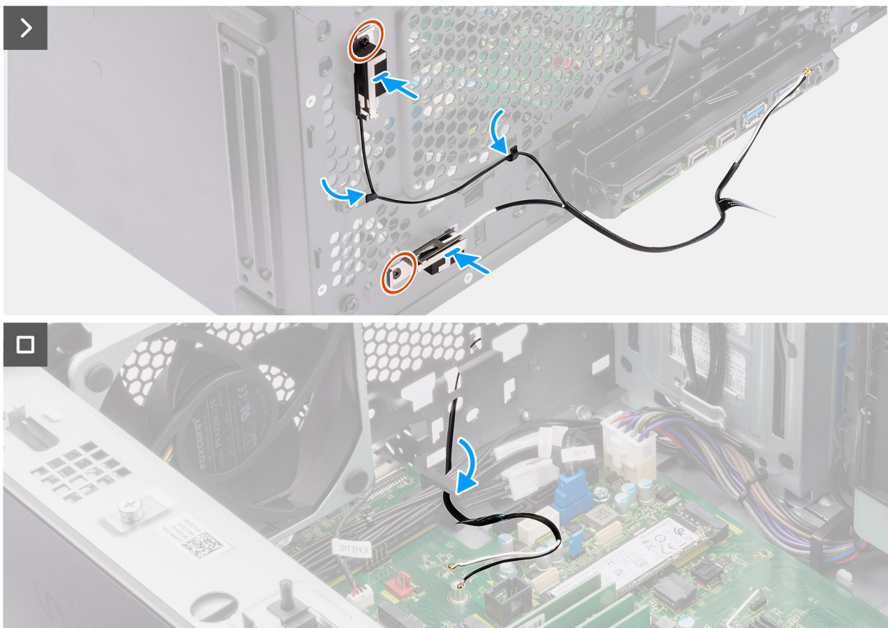
Figura 29. Installazione dell'antenna WLAN interna
