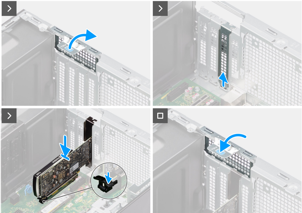
Figura 39. Installazione della scheda grafica
