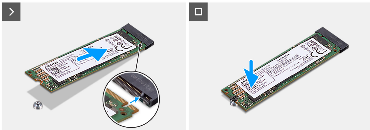
Figura 25. Installazione dell'unità SSD PCIe M.2 2280
