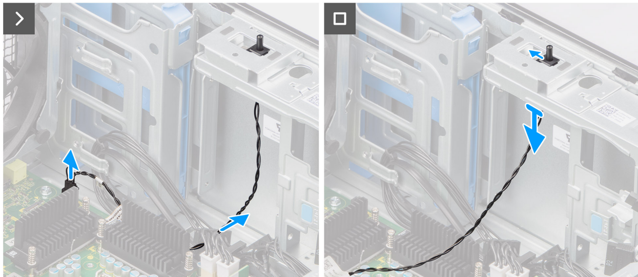
Figura 70. Rimozione dell'interruttore di intrusione
