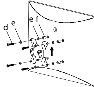
Per TV con retro curvo For curved back TV
