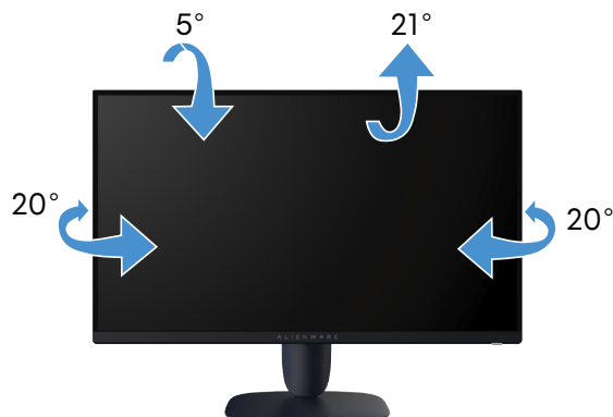
Figure 19. Regolazione inclinazione e oscillazione
