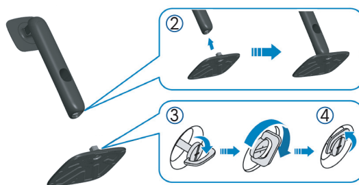
Figure 14. Collegare il supporto alla base
