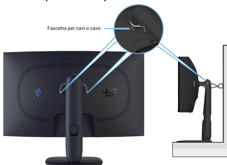
Figure 27. Protezione del monitor
