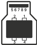
Figure 7. Porta upstream USB tipo B.
