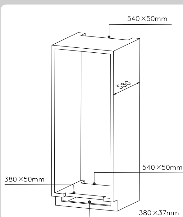
Maße der Schrankausschnitte
