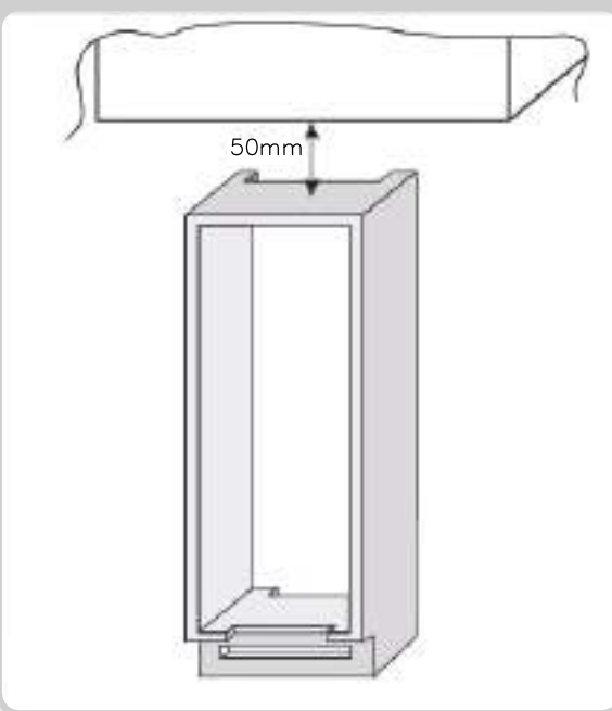
Erforderlicher Freiraum zwischen Gerät und Raumdecke.
