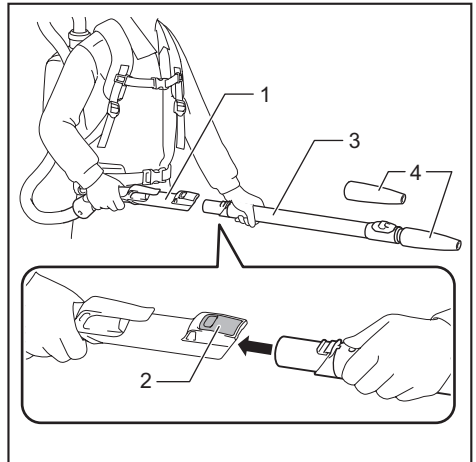
► 1. Ensemble de tuyau coudé 2. Bouton 3. Tube de rallonge coulissant 4. Buse amovible
