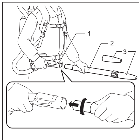
► 1. Ensemble de tuyau coudé 2. Tube de rallonge annulaire 3. Buse amovible
