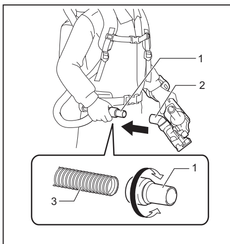
► 1. Manchon avant 2. Prise de collecte 3. Tuyau
