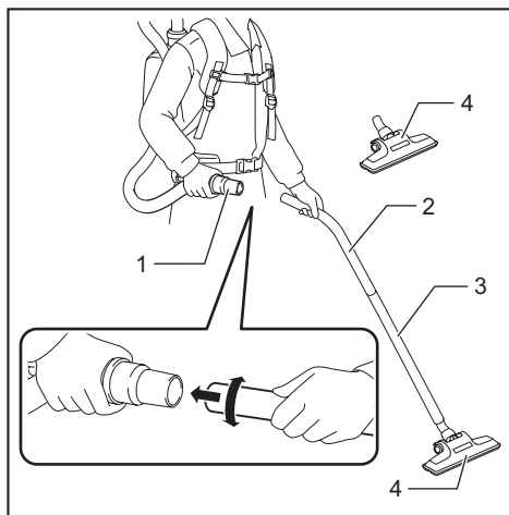
► 1. Manchon avant 38 2. Tuyau coudé en aluminium 3. Tuyau rectiligne en aluminium 4. Buse
