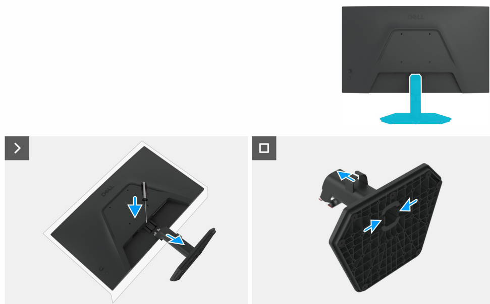
Figura 8. Rimozione del supporto
