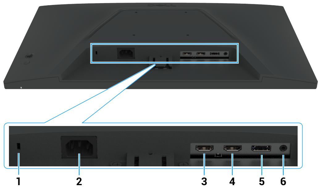
Figura 3. Vista dal basso
