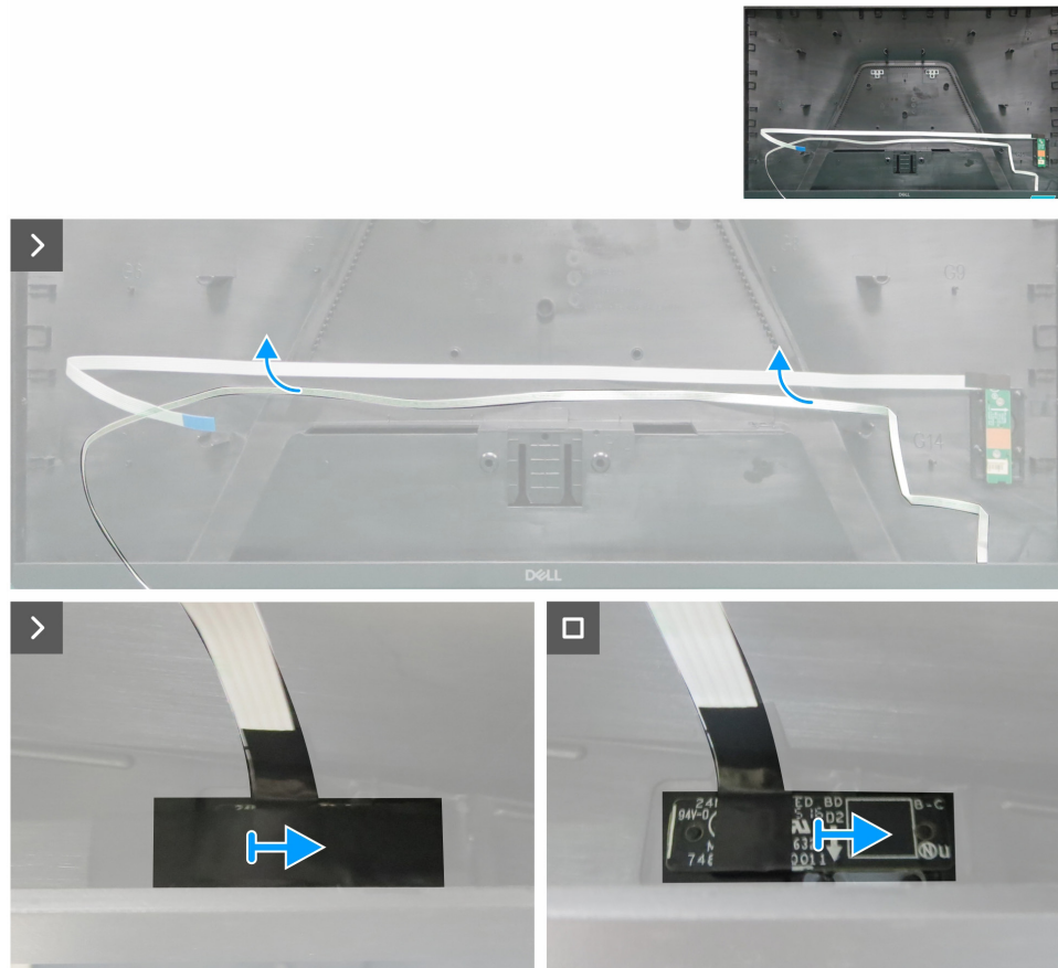
Figura 12. Rimozione della scheda LED
