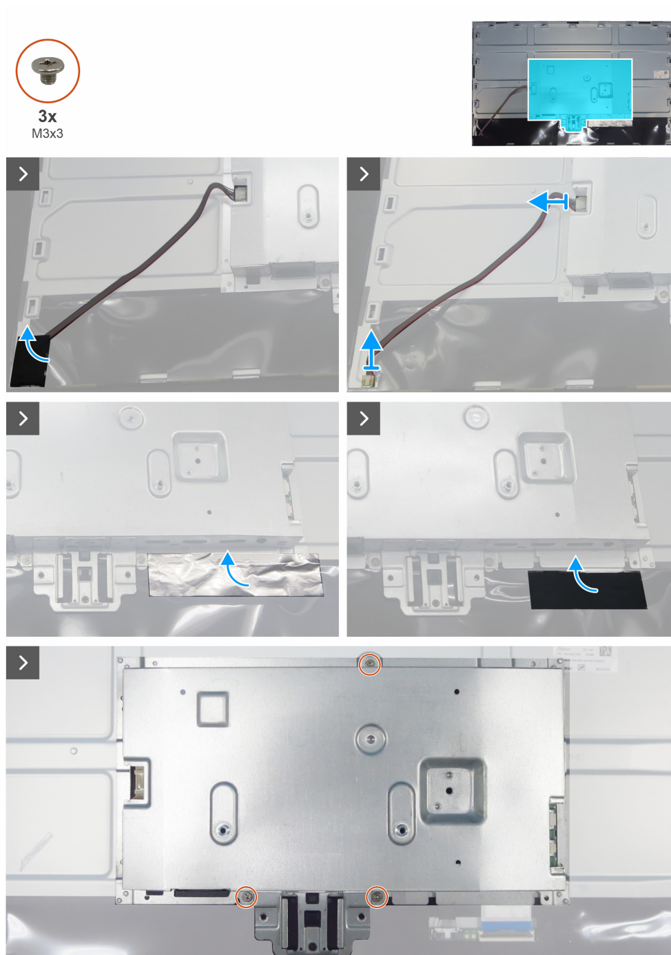
Figura 16. Rimozione del telaio principale
