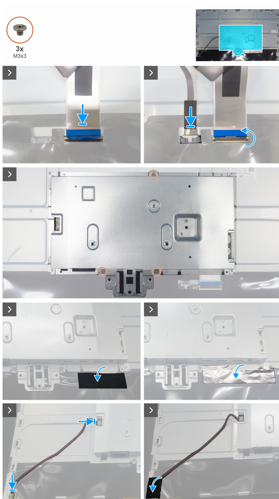
Figura 18. Installazione del telaio principale
