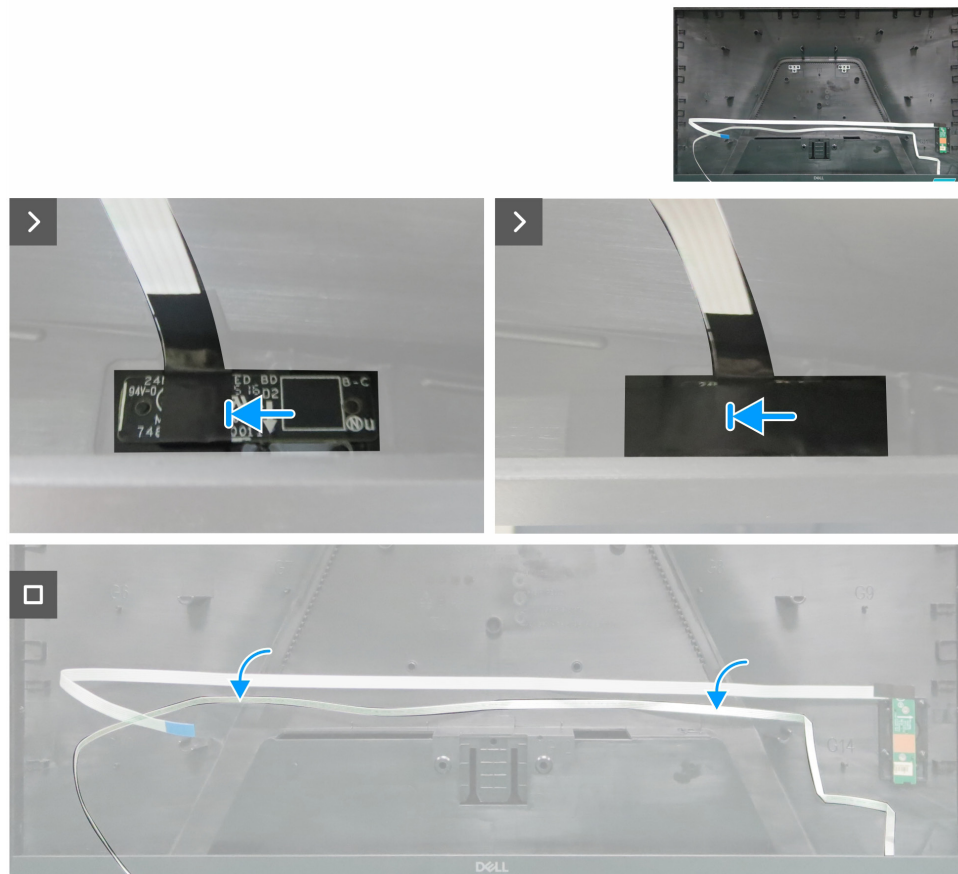
Figura 13. Installazione della scheda LED
