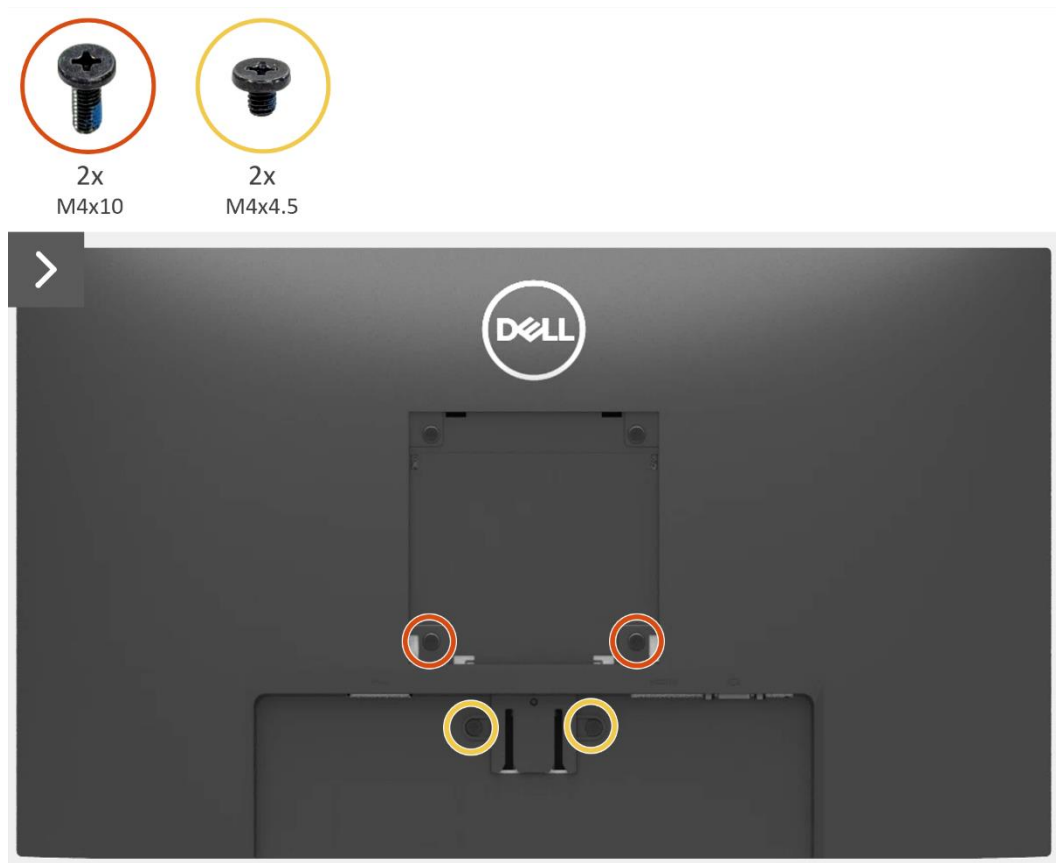
Figura 12. Rimozione del coperchio posteriore
