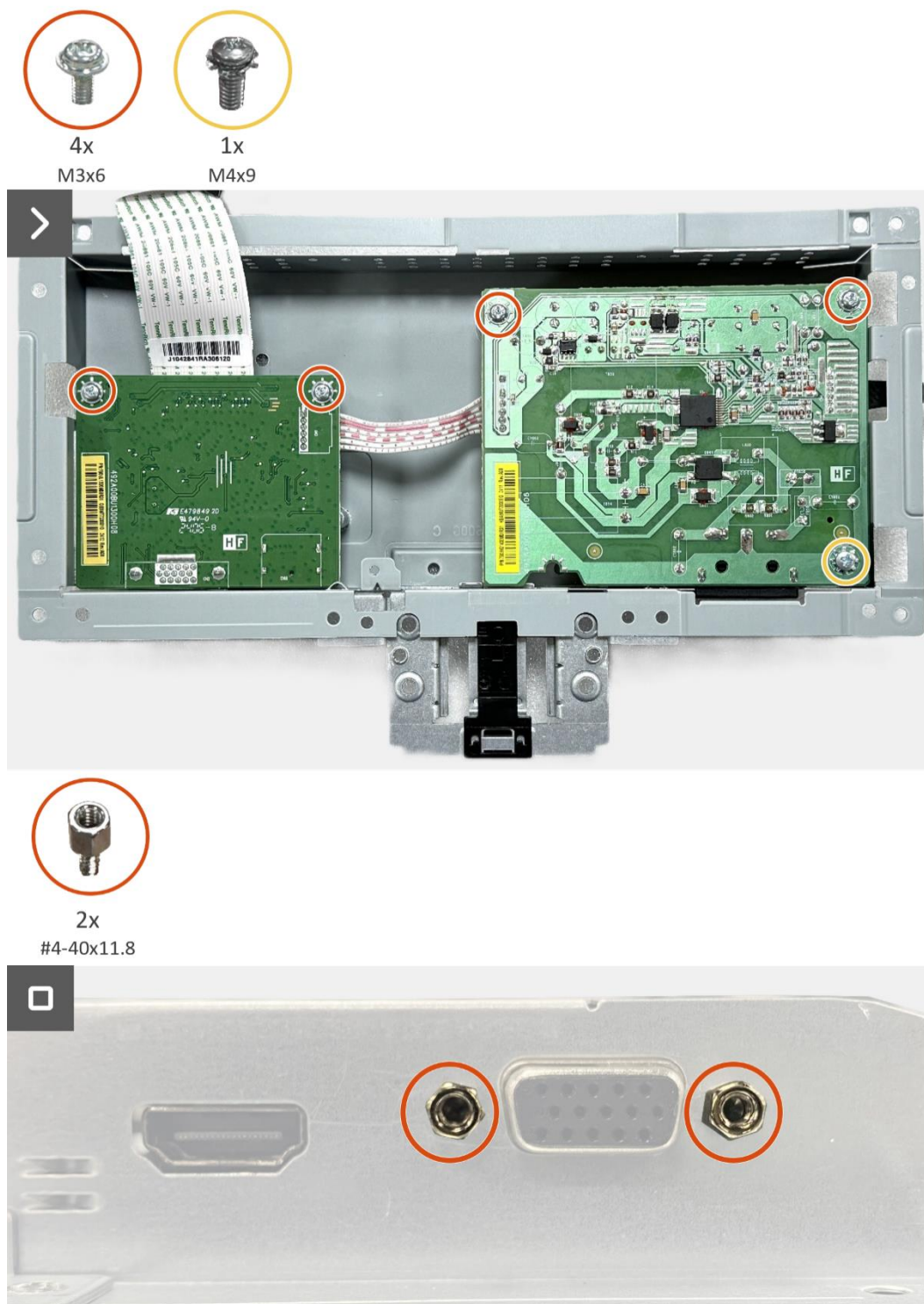
Figura 24. Installazione della scheda di interfaccia
