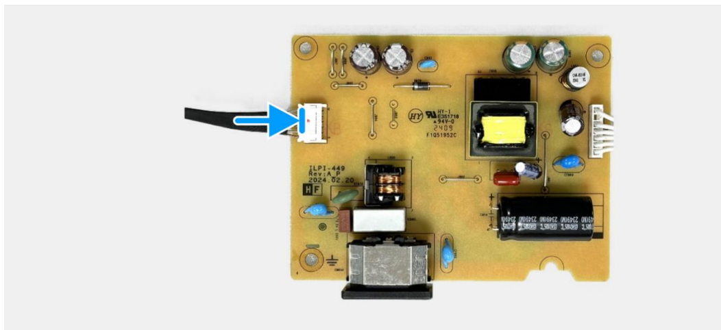
Figura 26. Installazione della scheda di alimentazione
