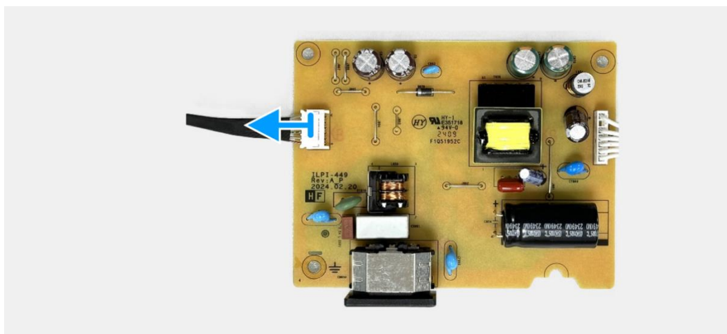
Figura 25. Rimozione della scheda di alimentazione
