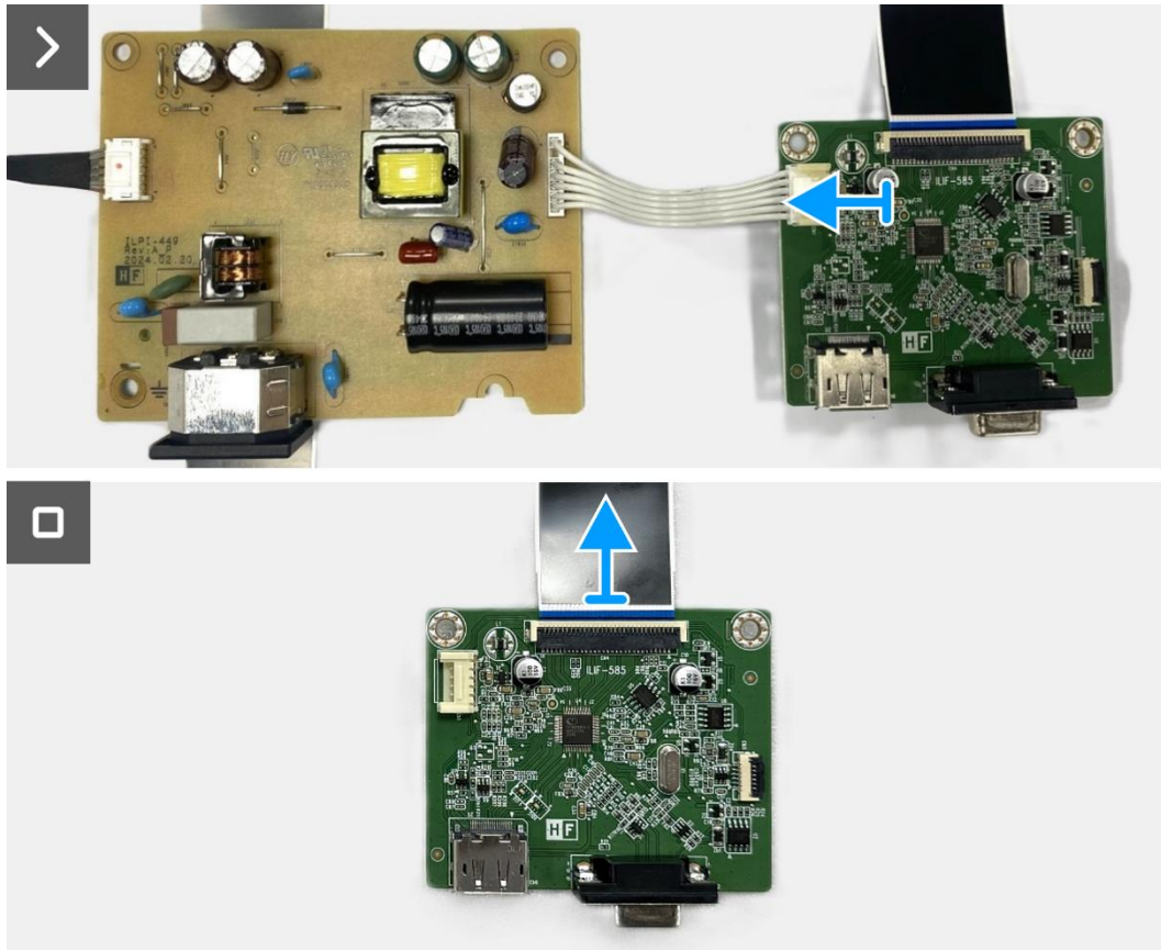
Figura 22. Rimozione della scheda di interfaccia
