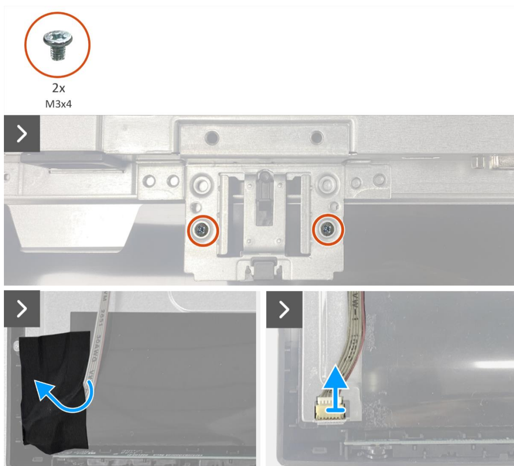
Figura 17. Rimozione del gruppo telaio
