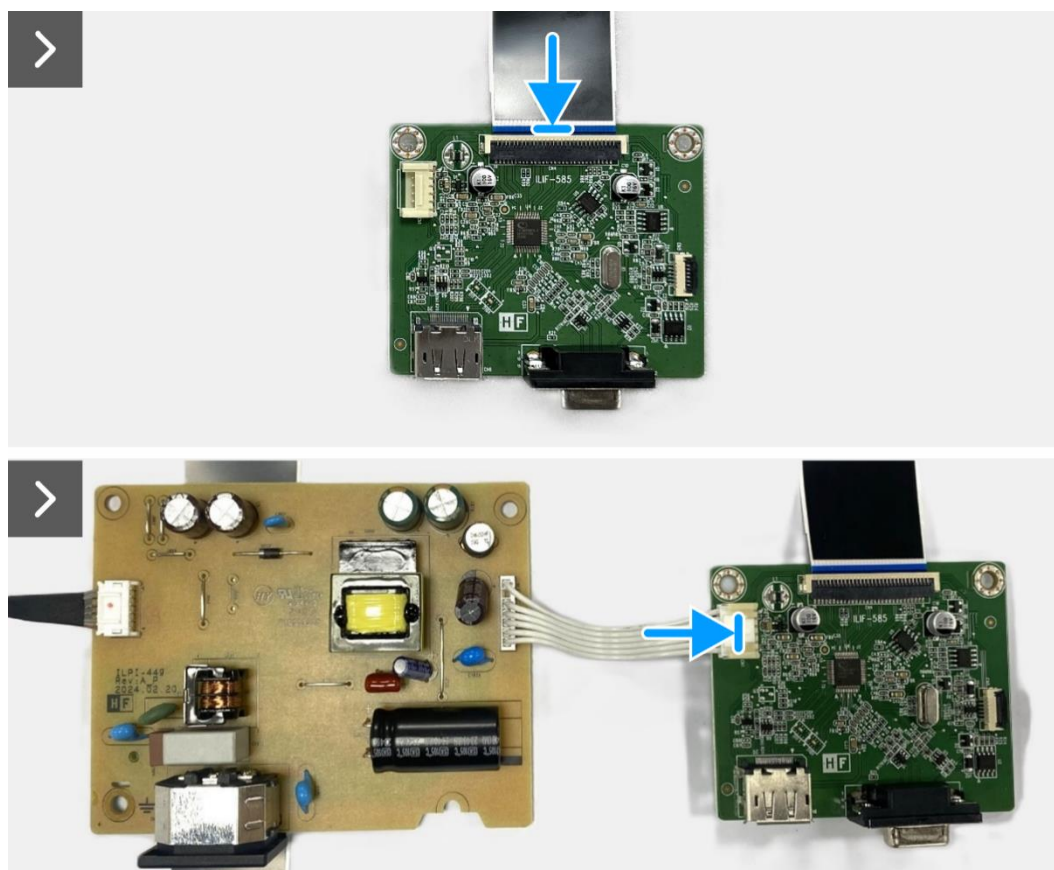
Figura 23. Installazione della scheda di interfaccia
