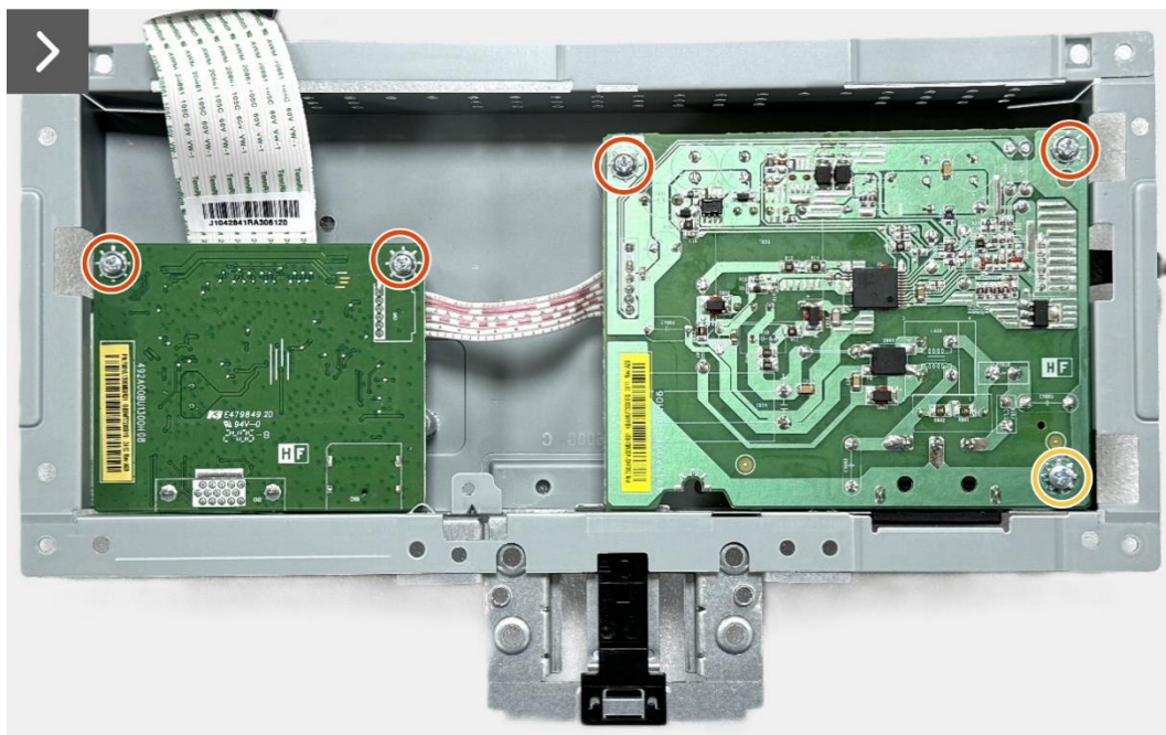
Figura 21. Rimozione della scheda di interfaccia
