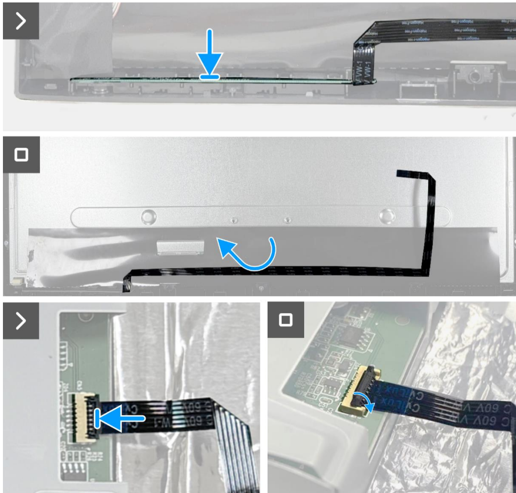
Figura 16. Installazione della scheda del tastierino
