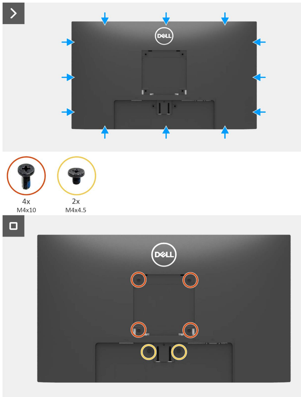
Figura 14. Installazione del coperchio posteriore
