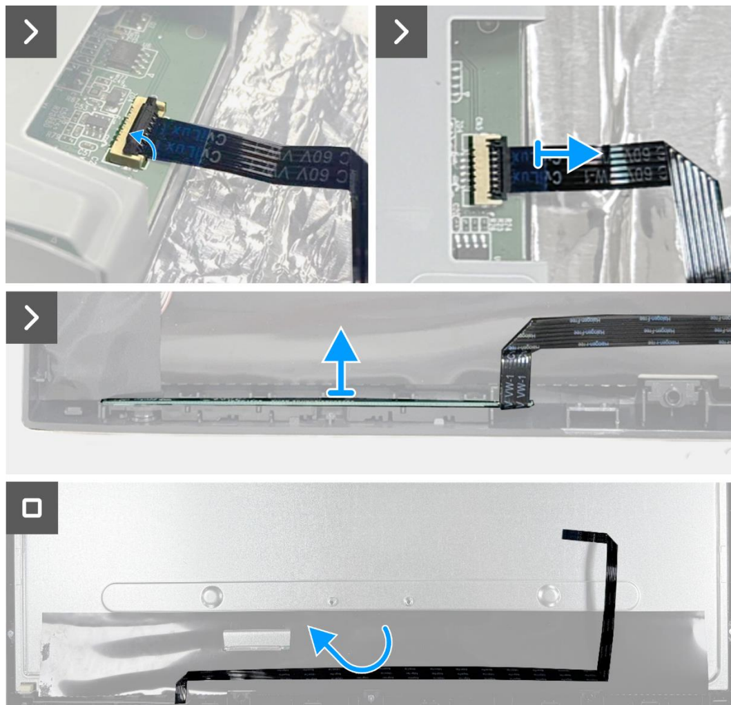
Figura 15. Rimozione della scheda del tastierino
