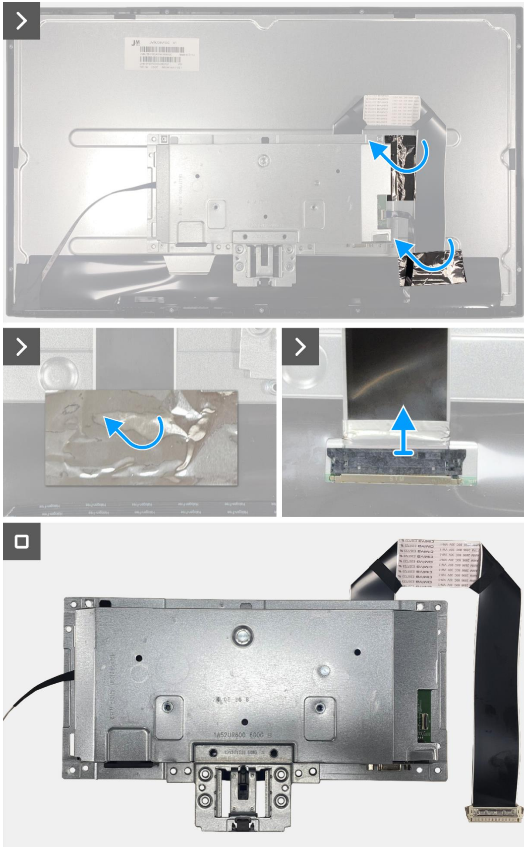
Figura 18. Rimozione del gruppo telaio
