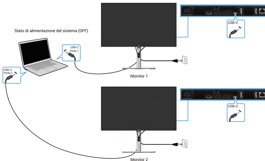
Figura 50. Alimentazione USB-C 90 W per Accendere in modalità Spento
