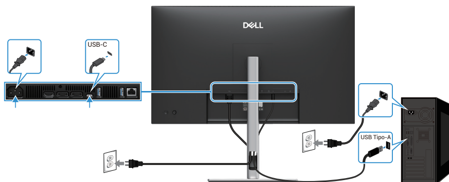
Figura 30. Collegamento del cavo USB Tipo-C a Tipo-A
