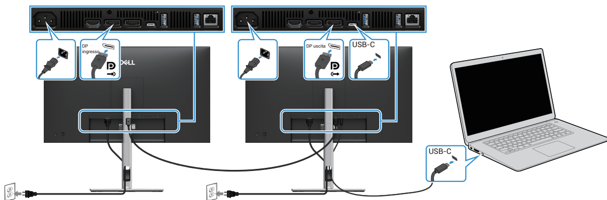
Figura 33. Collegamento del monitor per la funzione USB-C MST
