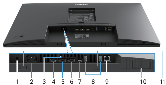
Figura 5. Vista dal basso senza supporto per monitor
