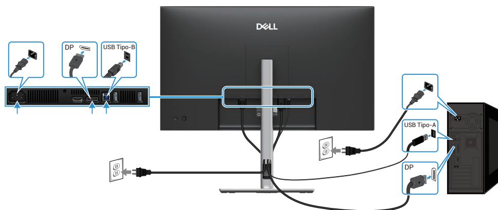
Figura 28. Collegamento del cavo DisplayPort e USB
