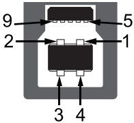
Figura 10. Connettore upstream USB 5Gbps Tipo-B
