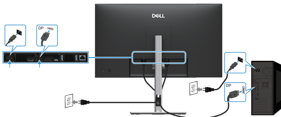
Figura 27. Collegamento del cavo DisplayPort
