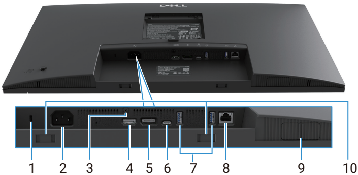
Figura 6. Vista dal basso senza supporto per monitor
