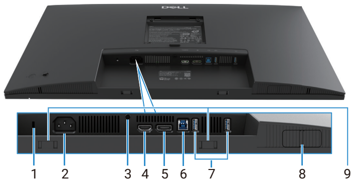
Figura 4. Vista dal basso senza supporto per monitor
