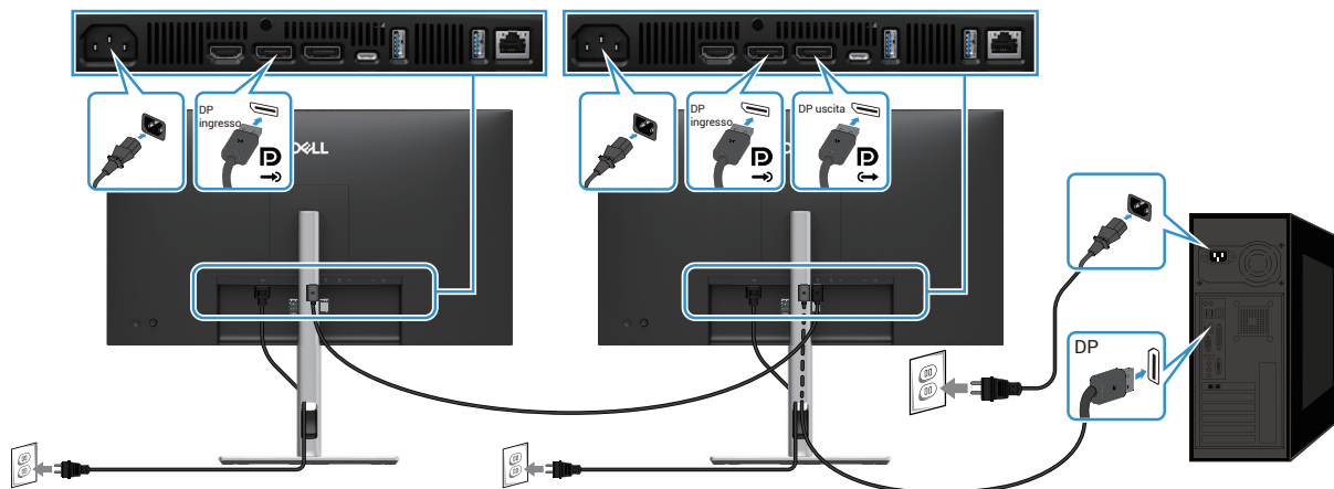
Figura 32. Collegamento del monitor per la funzione DP MST
