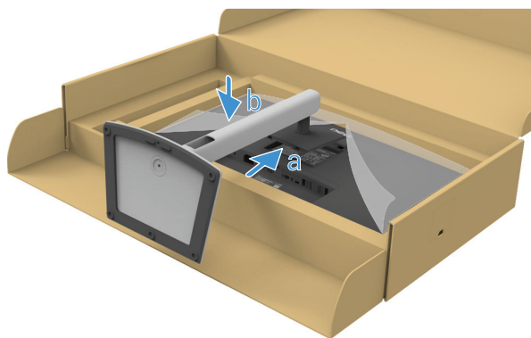
Figura 22. Fissare il supporto al monitor
