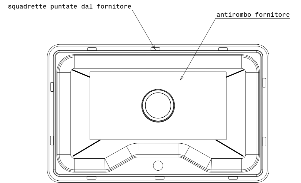
Vista da sotto Scala: 1:8
