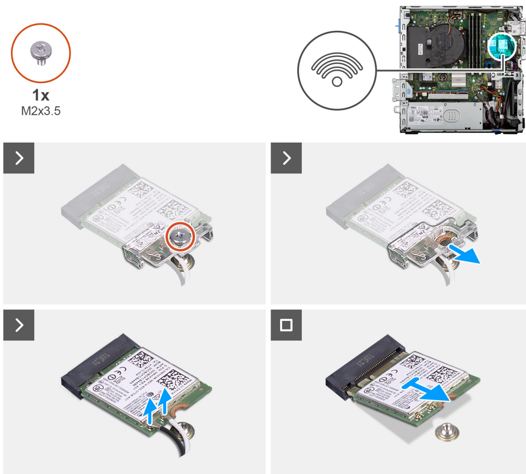
Figura 29. Rimozione della scheda wireless
