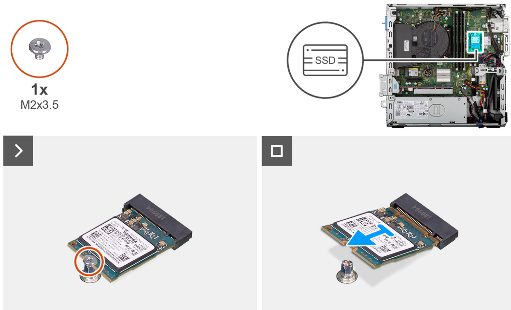
Figura 19. Rimozione dell'unità SSD M.2 2230
