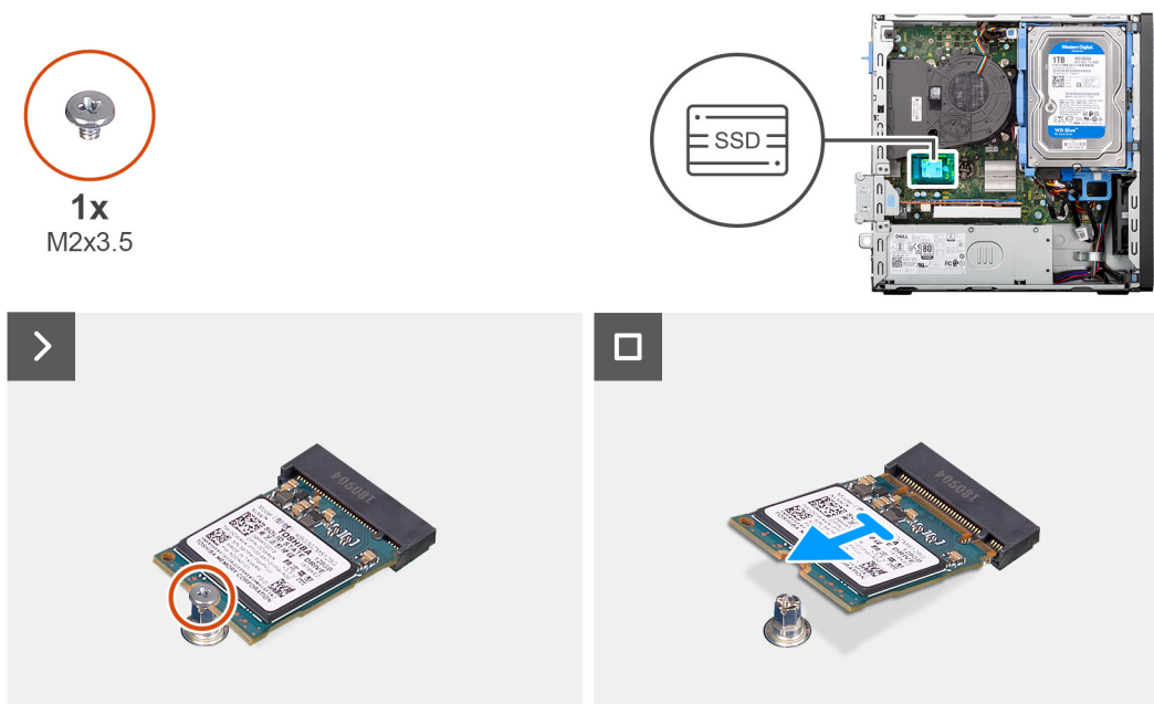
Figura 17. Rimozione dell'unità SSD M.2 2230
