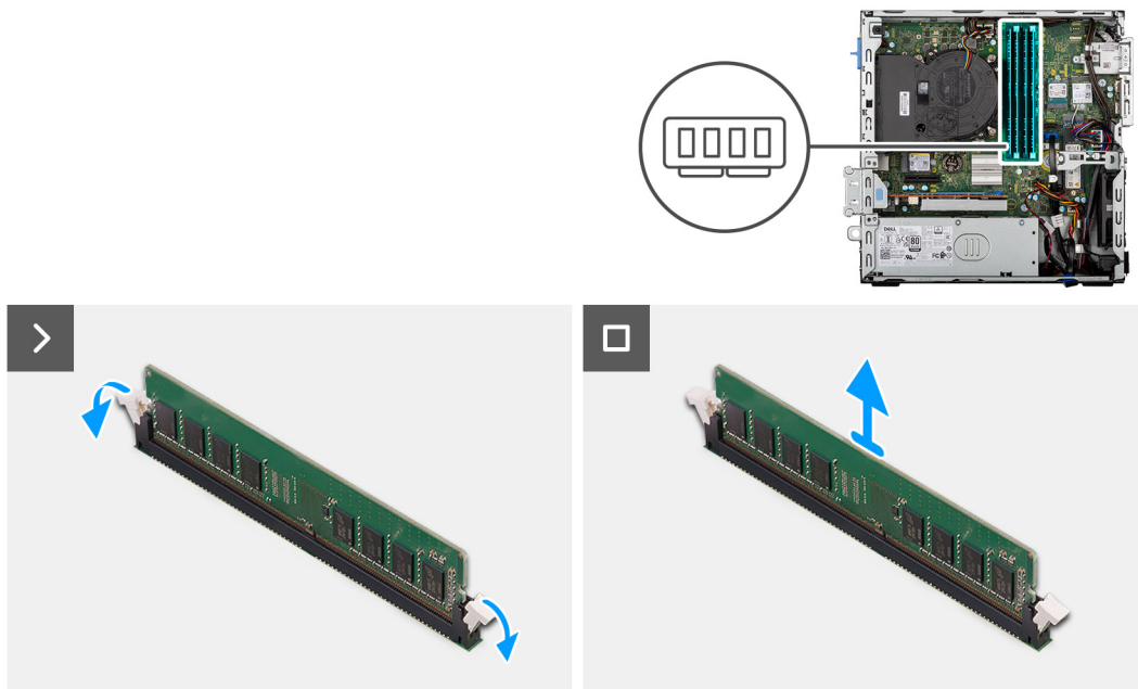
Figura 15. Rimozione della memoria
