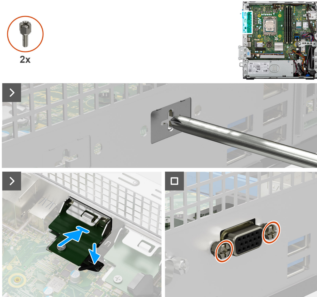
Figura 61. Installazione del modulo VGA
