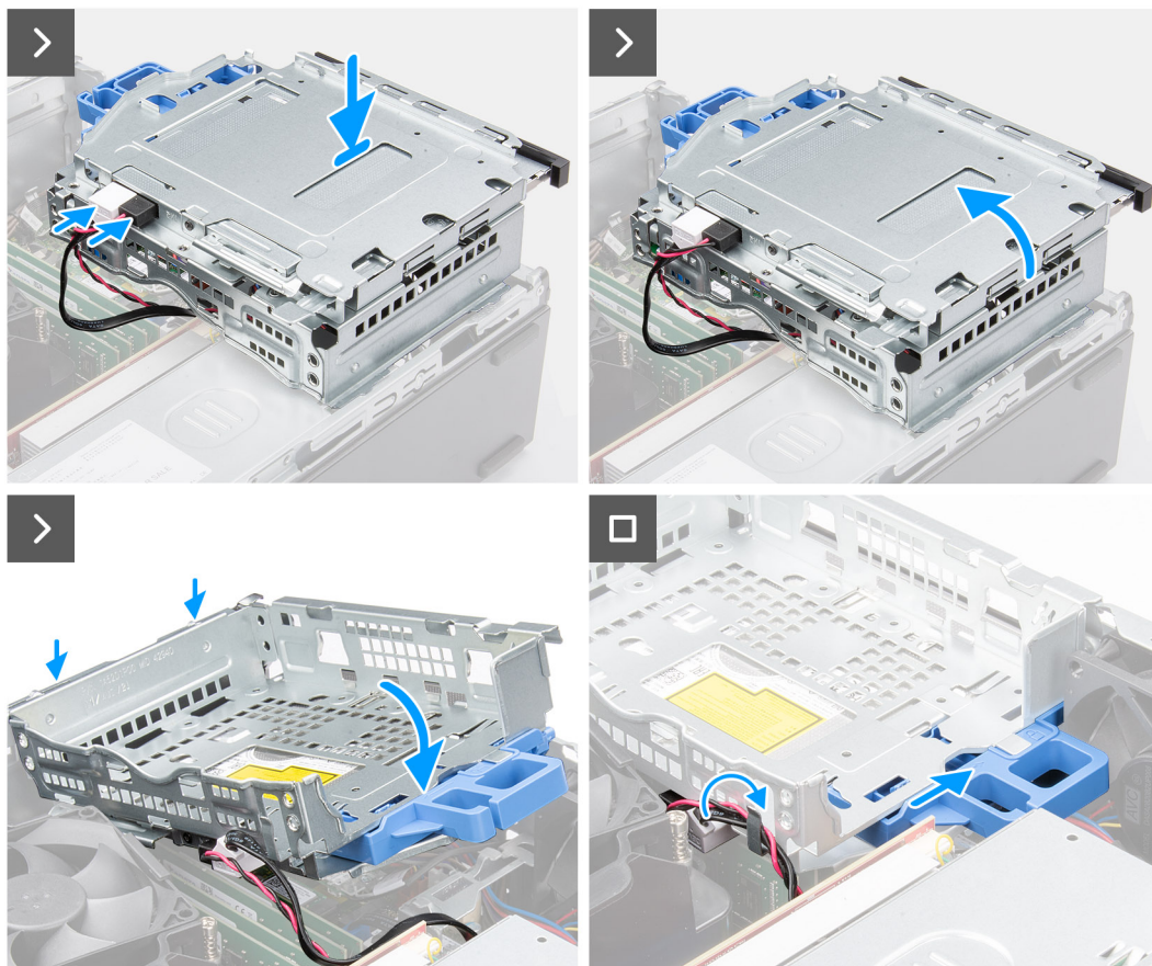
Figura 12. Installazione della gabbia del disco rigido
