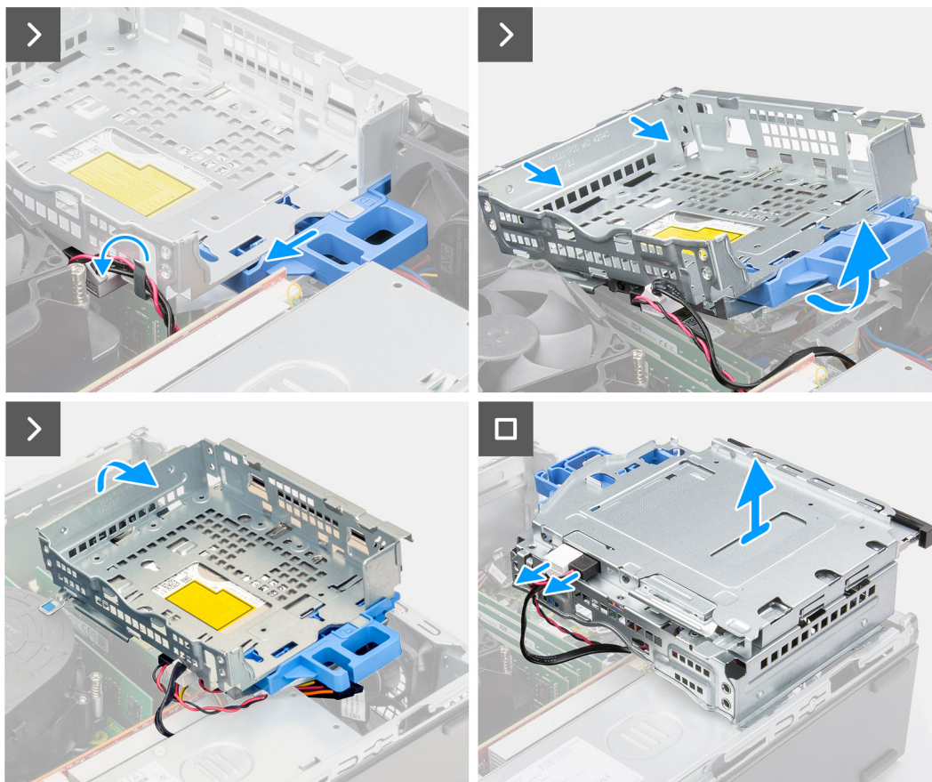
Figura 11. Rimozione della gabbia del disco rigido
