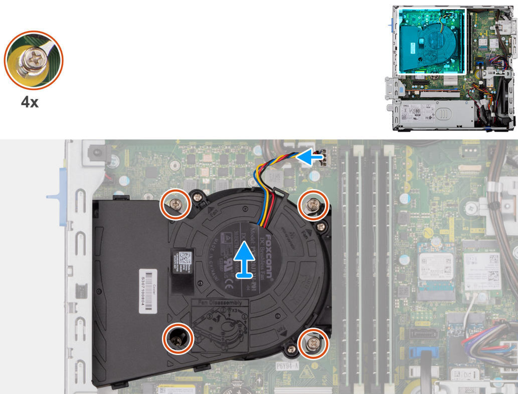
Figura 50. Rimozione del gruppo ventola del processore e dissipatore di calore
