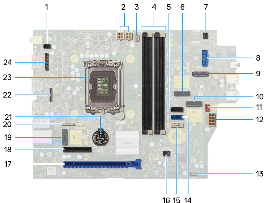
Figura 64. Panoramica della scheda di sistema
