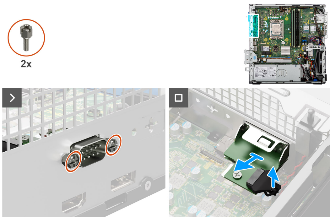
Figura 54. Rimozione del modulo seriale
