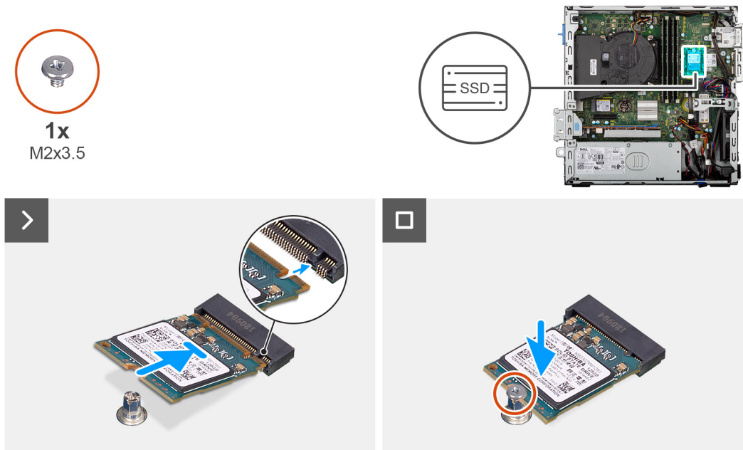
Figura 20. Installazione delle unità SSD M.2 2230 nello slot 1
