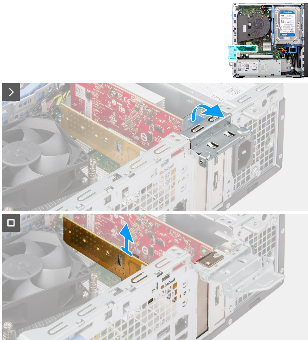
Figura 23. Rimozione della scheda Dell Ultra Speed Drive Gen3
