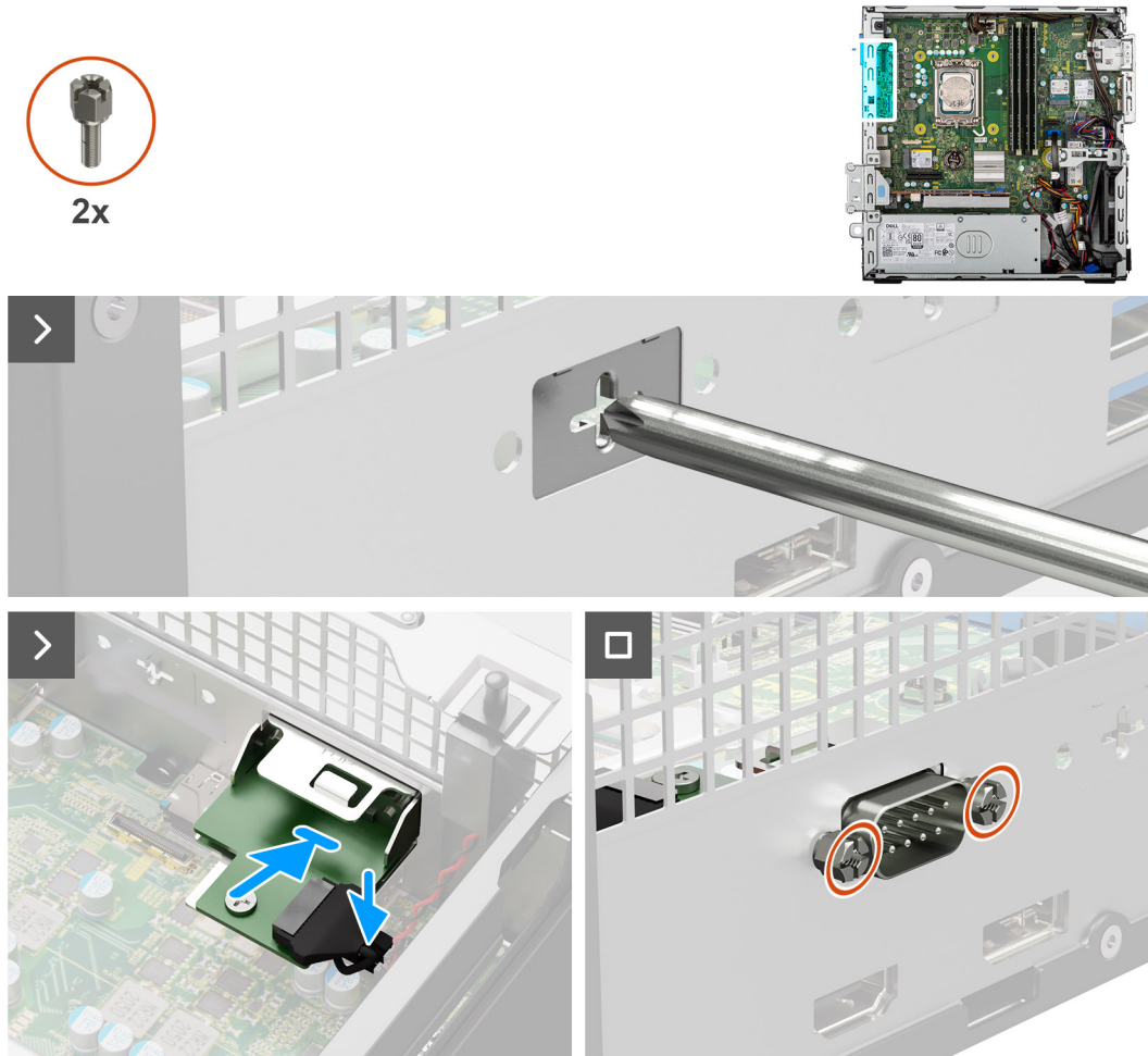
Figura 55. Installazione del modulo seriale
