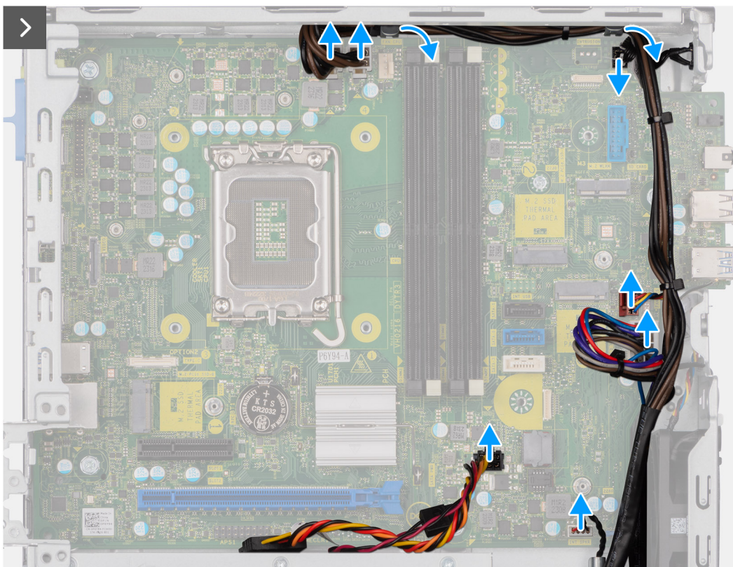
Figura 66. Rimozione della scheda di sistema
