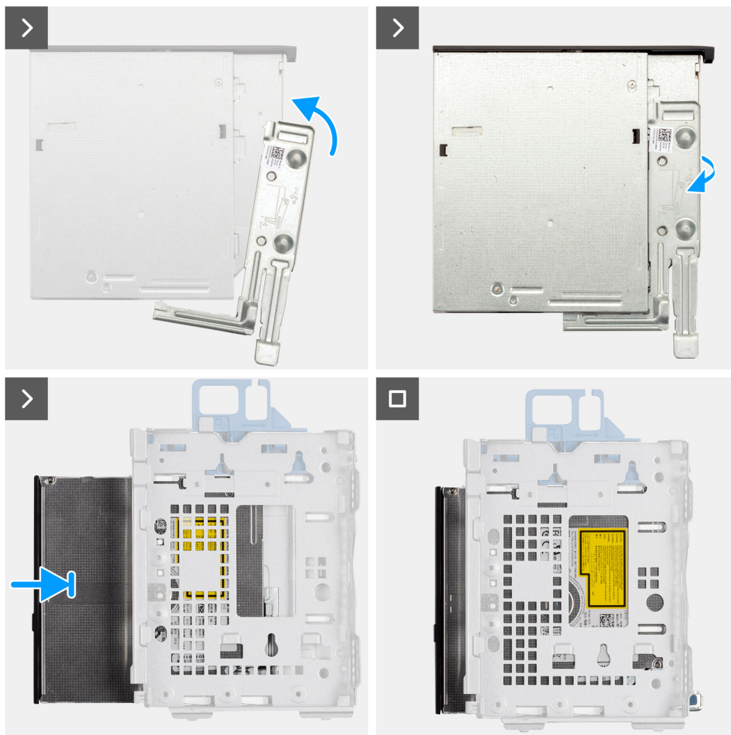
Figura 14. Installazione dell'unità ottica
