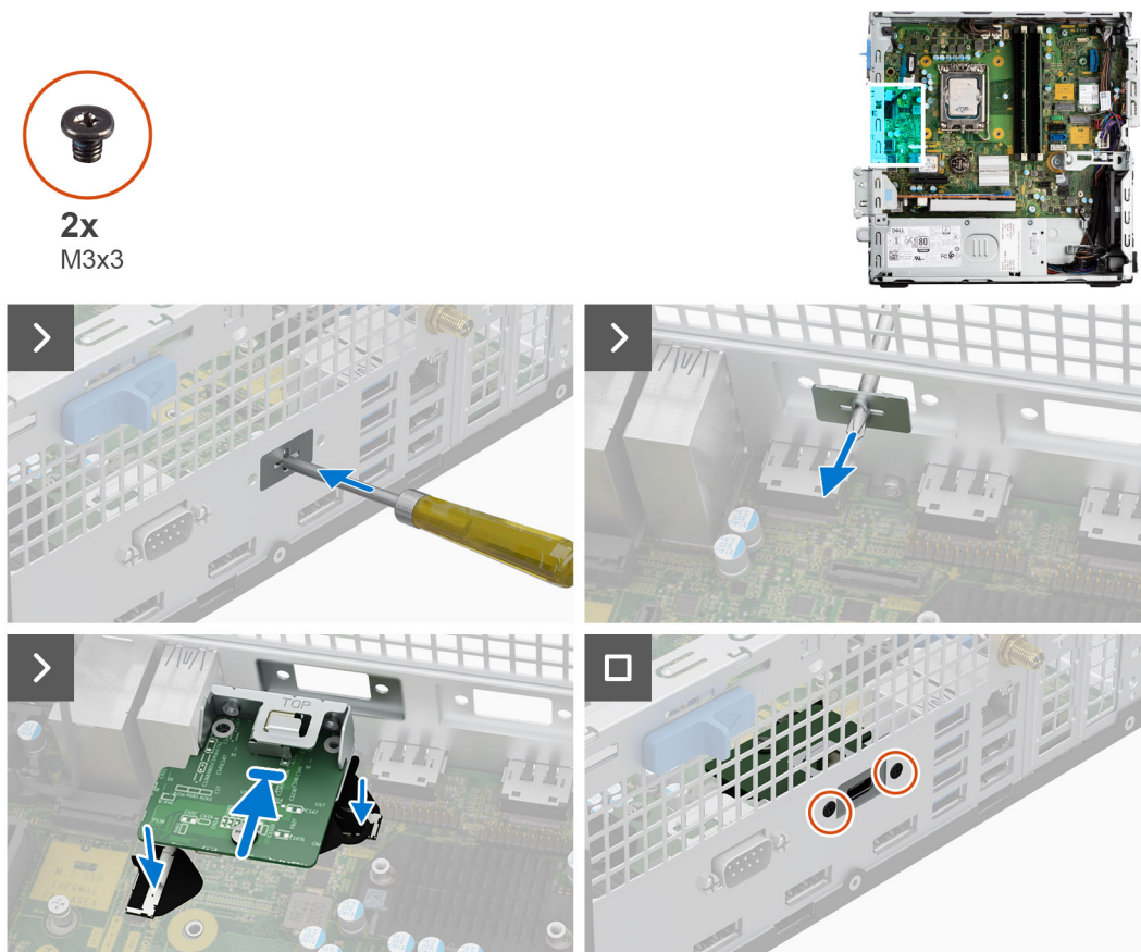
Figura 63. Installazione del modulo Type-C
