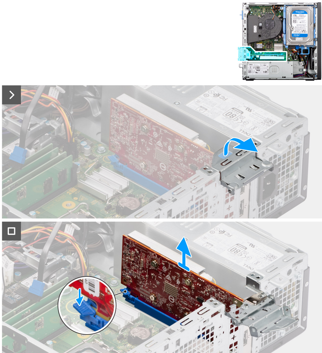
Figura 33. Rimozione della scheda grafica
