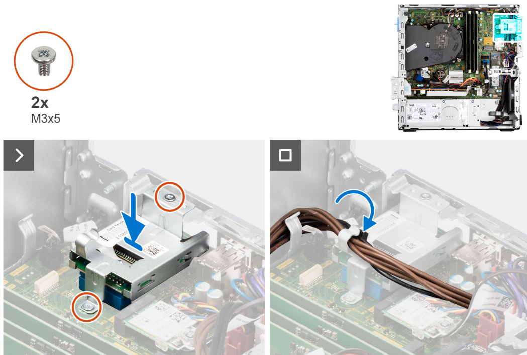
Figura 32. Installazione del lettore di schede multimediali
