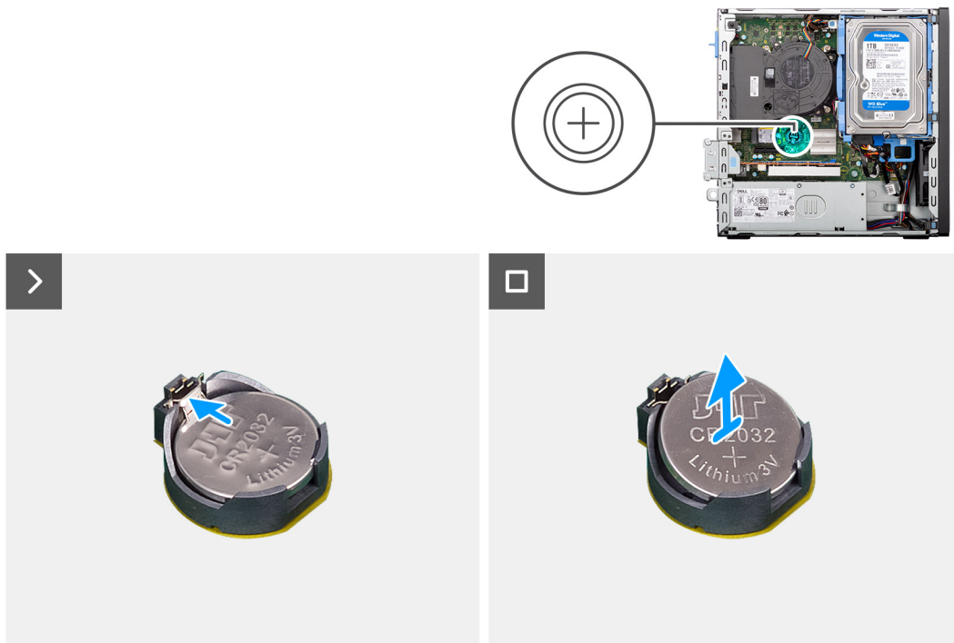
Figura 5. Rimozione della batteria a bottone
