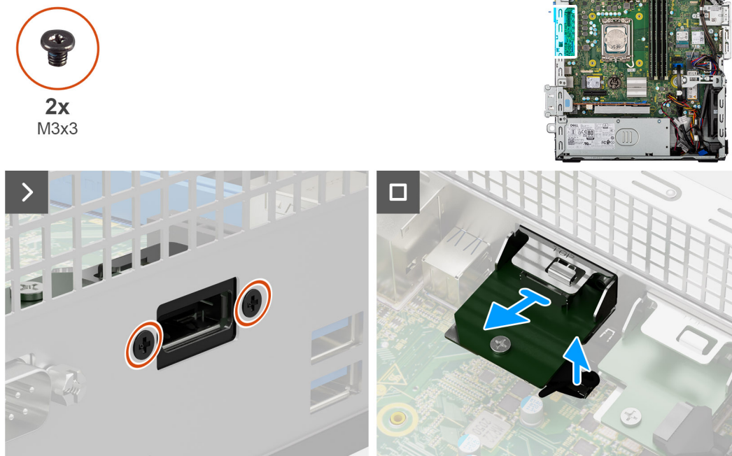
Figura 56. Rimozione del modulo DisplayPort
