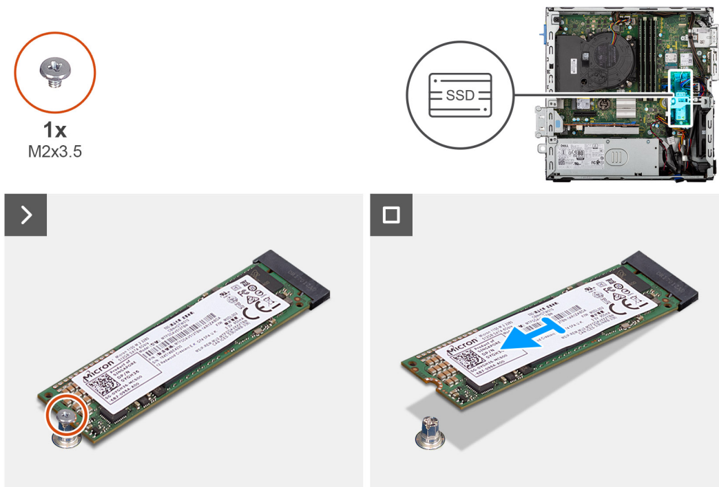
Figura 21. Rimozione dell'unità SSD M.2 2280
