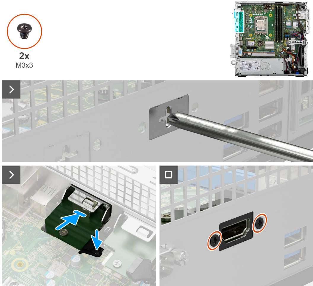
Figura 59. Installazione del modulo HDMI
