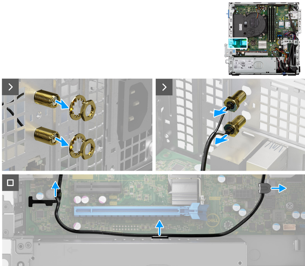
Figura 46. Rimozione del modulo antenna SMA esterna
