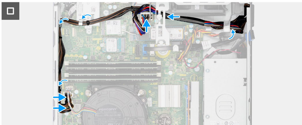
Figura 49. Installazione dell'unità di alimentazione
