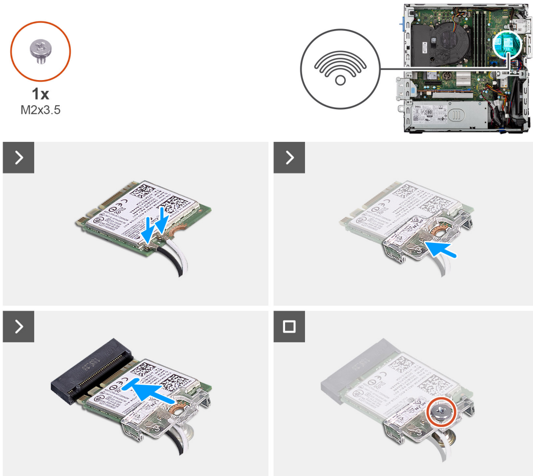
Figura 30. Installazione della scheda wireless
