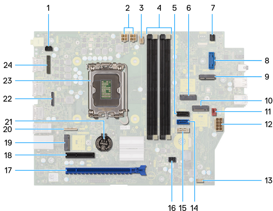
Figura 69. Panoramica della scheda di sistema
