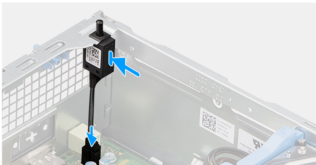
Figura 38. Installazione dello switch antintrusione
