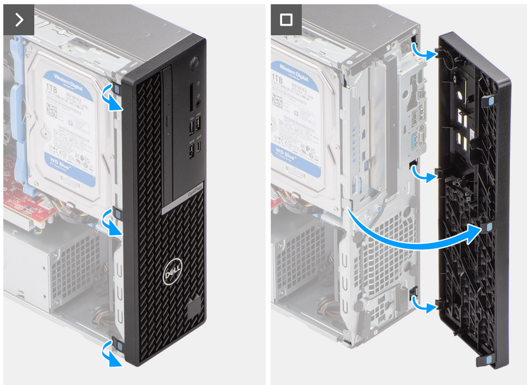
Figura 7. Rimozione del pannello anteriore
