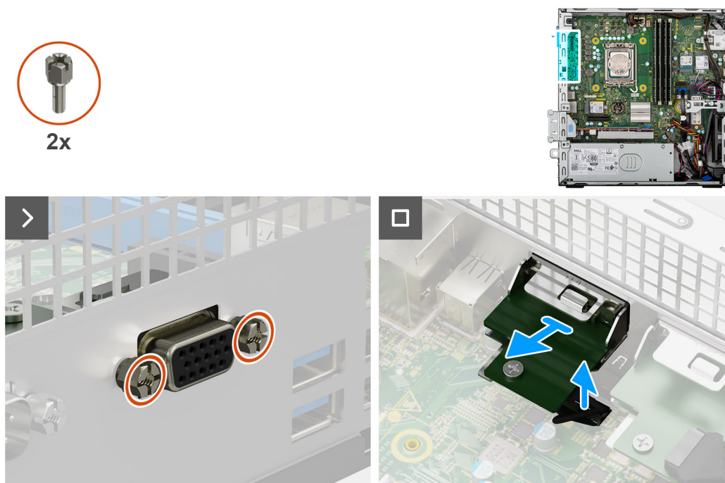
Figura 60. Rimozione del modulo VGA
