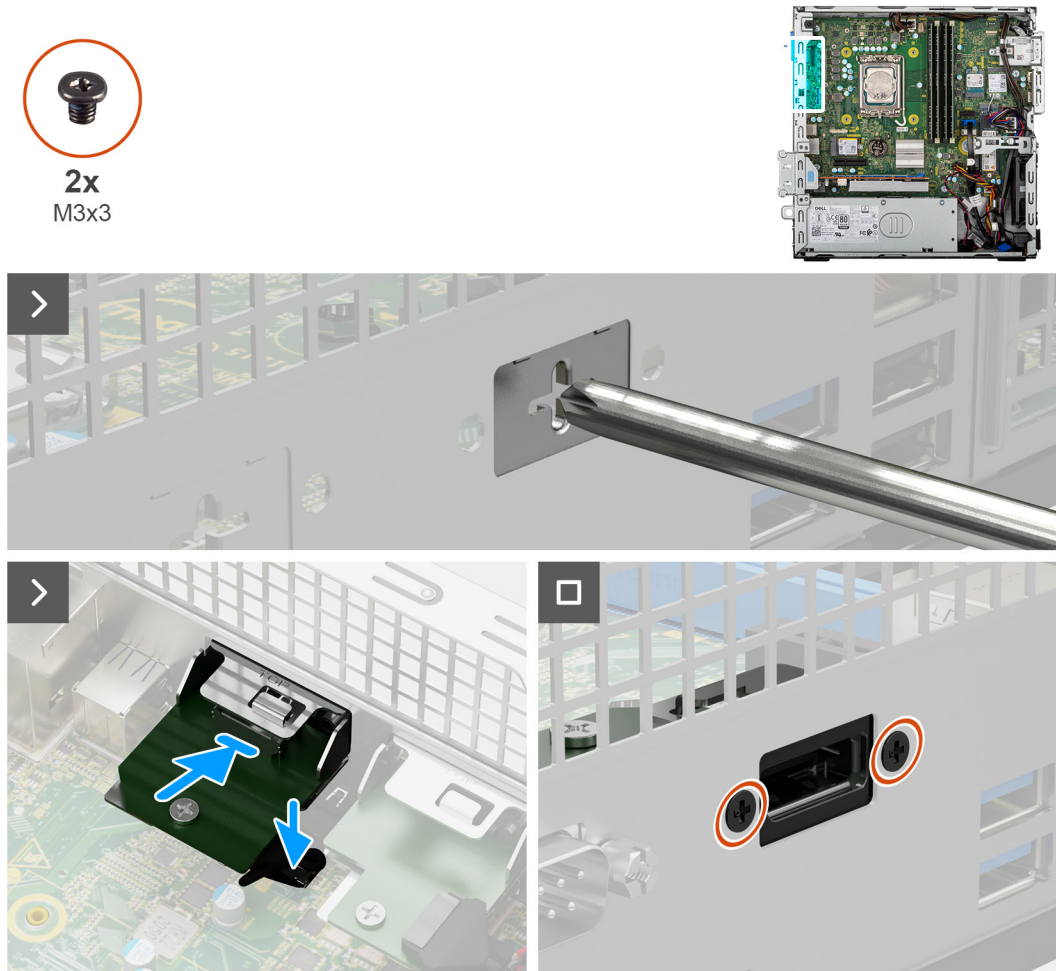
Figura 57. Installazione del modulo DisplayPort
