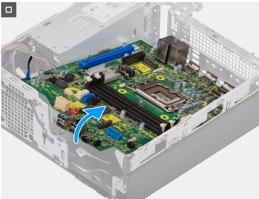
Figura 68. Rimozione della scheda di sistema
