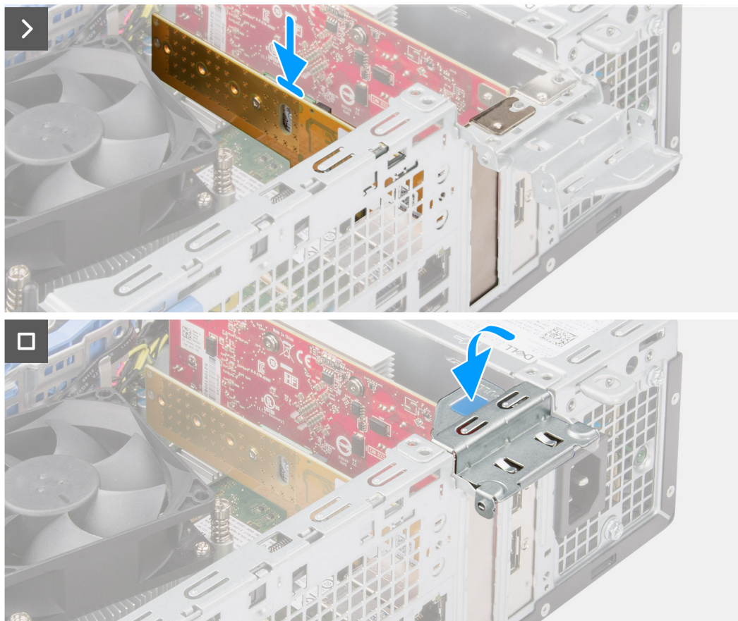
Figura 28. Installazione della scheda Dell Ultra Speed Drive Gen3
