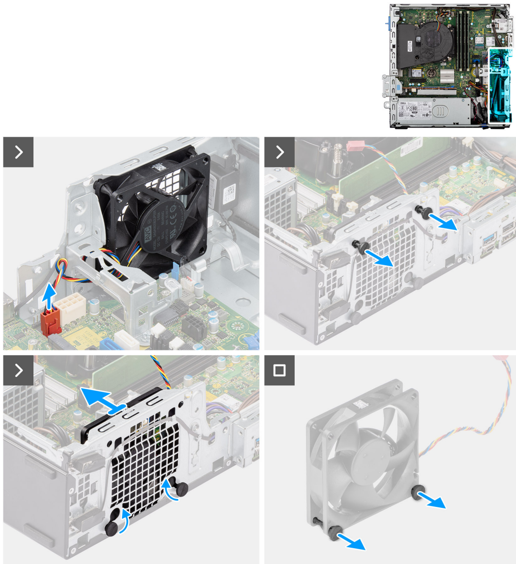
Figura 41. Rimozione della ventola di sistema
