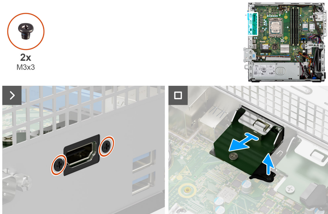
Figura 58. Rimozione del modulo HDMI
