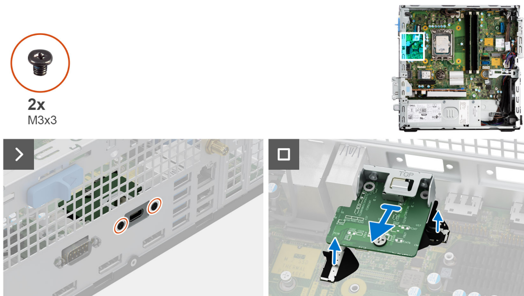
Figura 62. Rimozione del modulo Type-C
