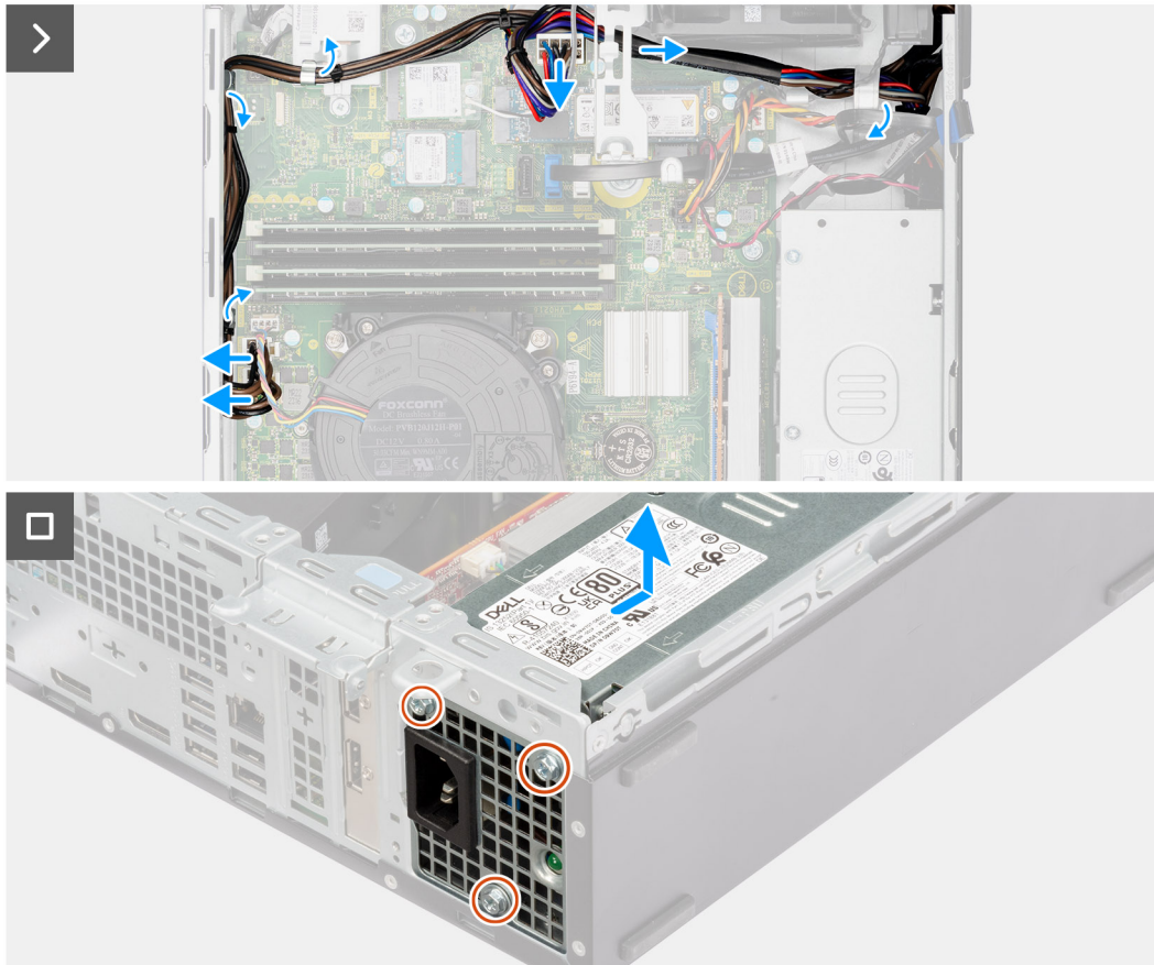
Figura 48. Rimozione dell'unità di alimentazione
