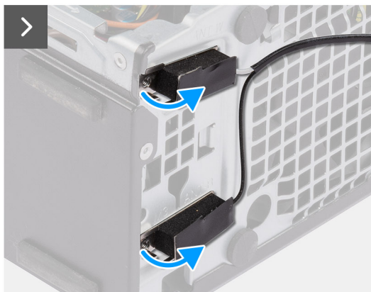
Figura 43. Rimozione del modulo dell'antenna interna
