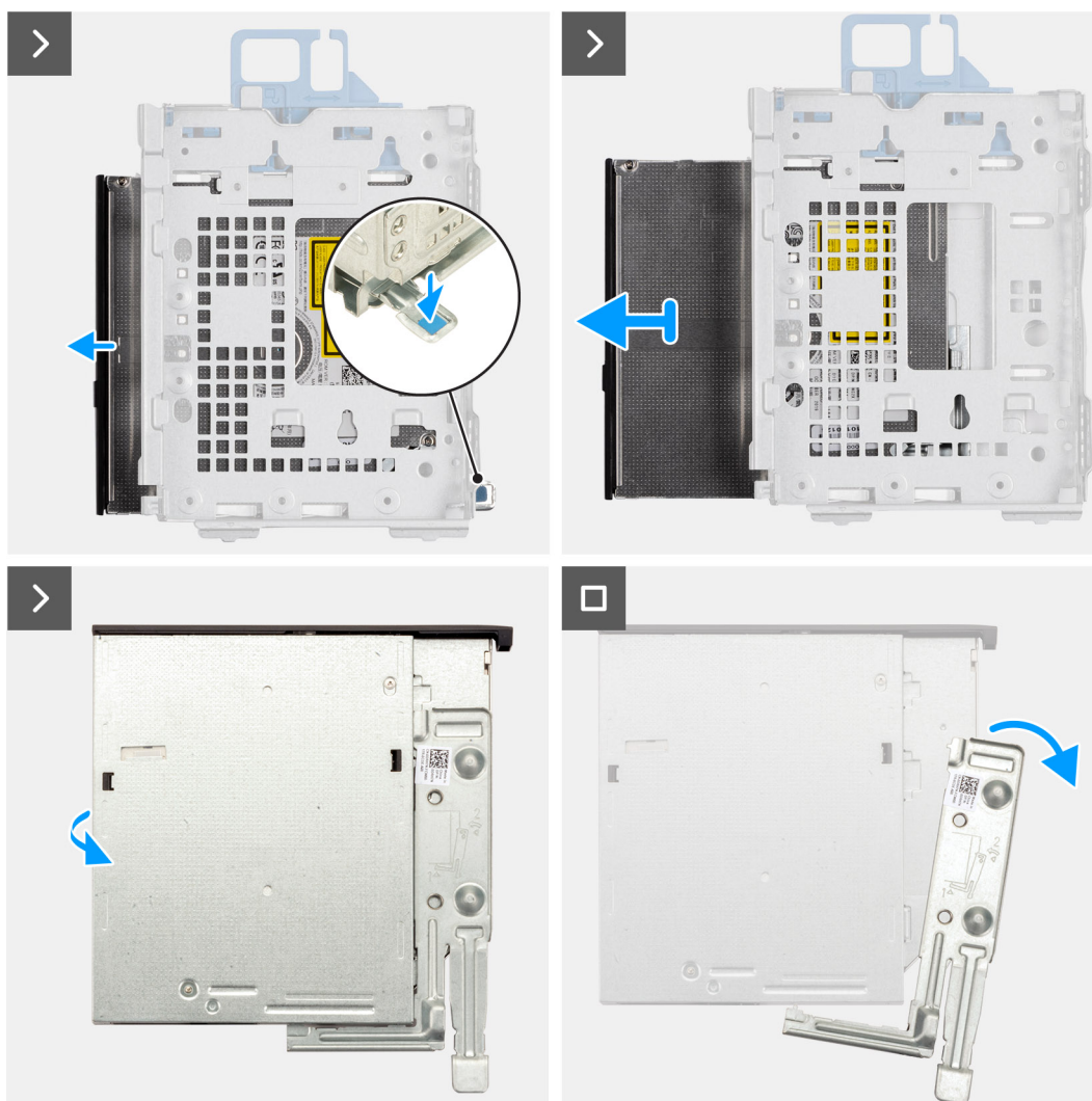
Figura 13. Rimozione dell'unità ottica
