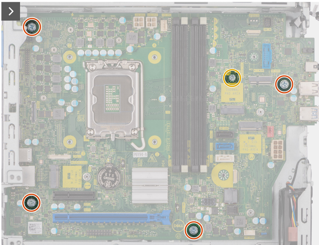
Figura 71. Installazione della scheda di sistema
