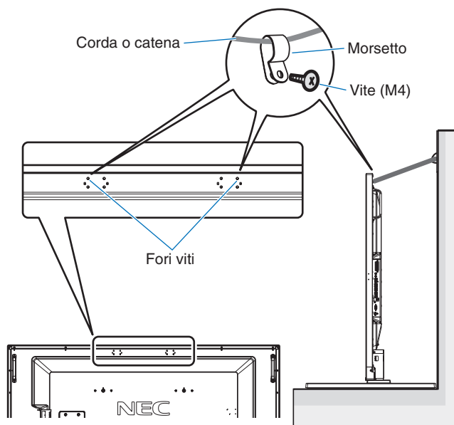
Senza staffe con bulloni a occhiello
