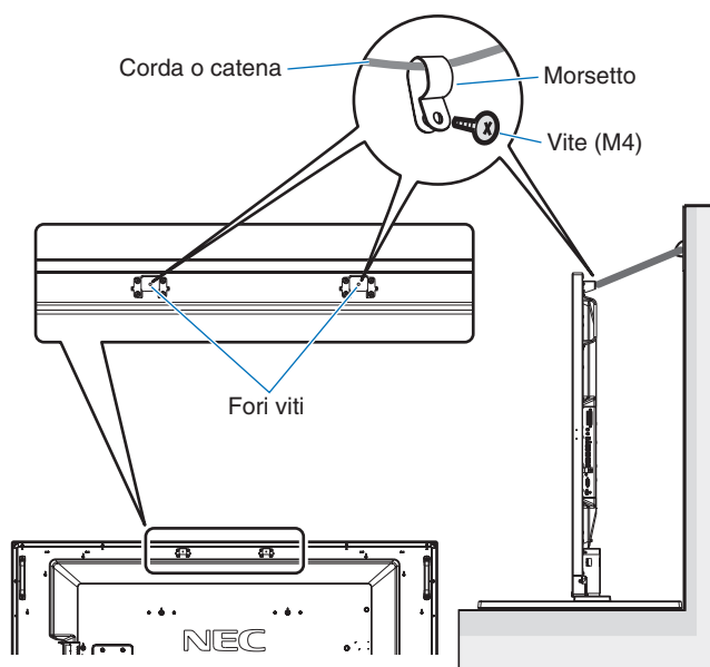
Con staffe con bulloni a occhiello
