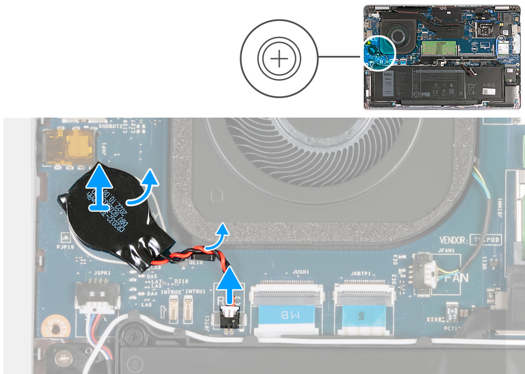
Figura 20. Rimozione della batteria a bottone
