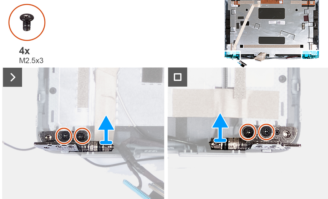
Figura 47. Rimozione dei cardini del display
