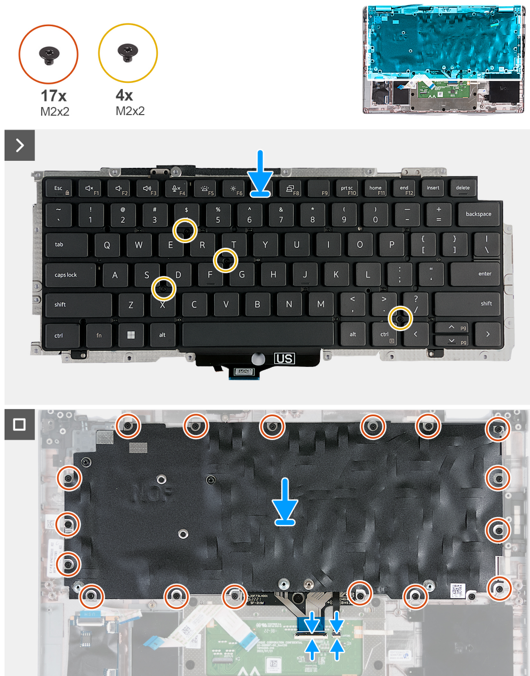
Figura 62. Installazione della tastiera
